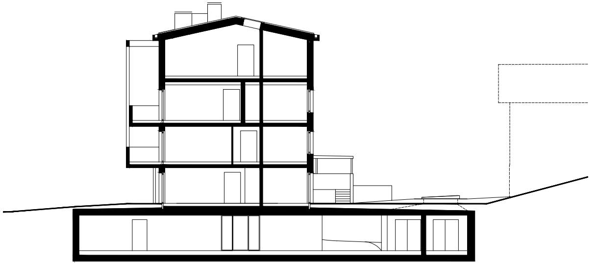
SCHNITT
