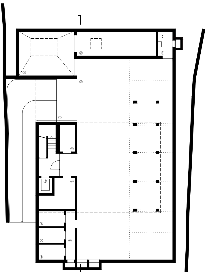
UNTERGESCHOSS
