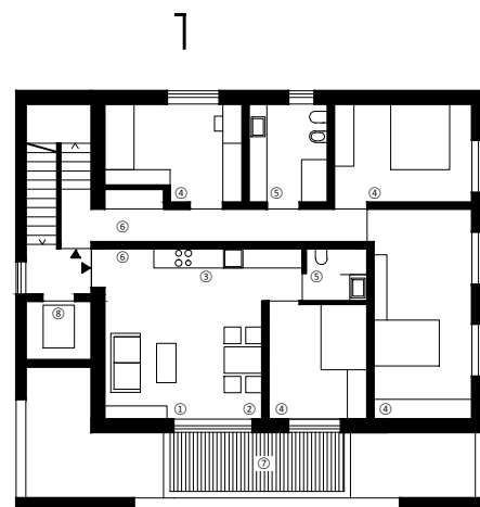
2. OBERGESCHOSS
