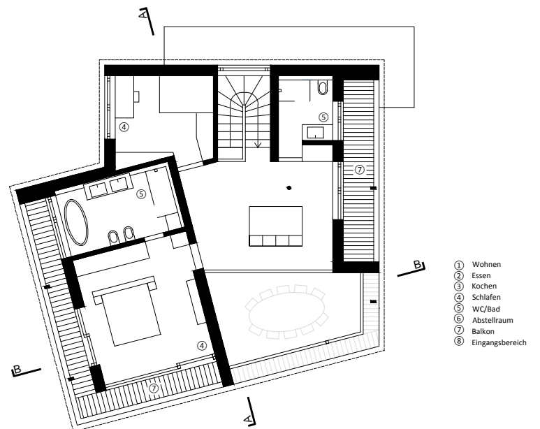
DACHGESCHOSS
