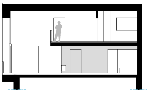
SCHNIITT A-A
