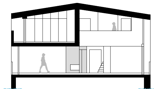
SCHNIITT B-B
