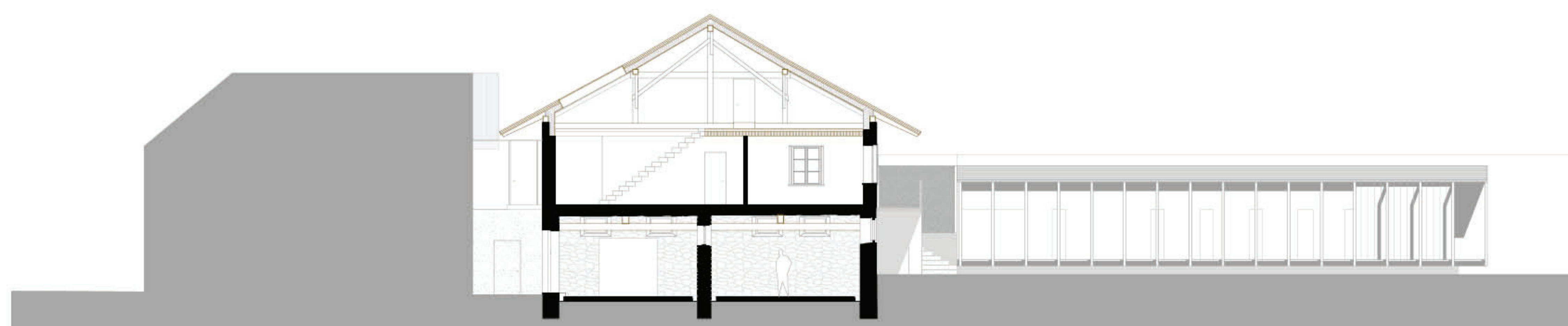
SCHNITT HOFSTELLE
