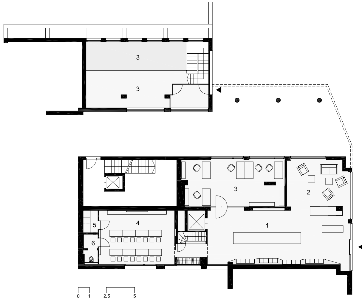
VINOTHEK VINUM, Bozen M 1:200
