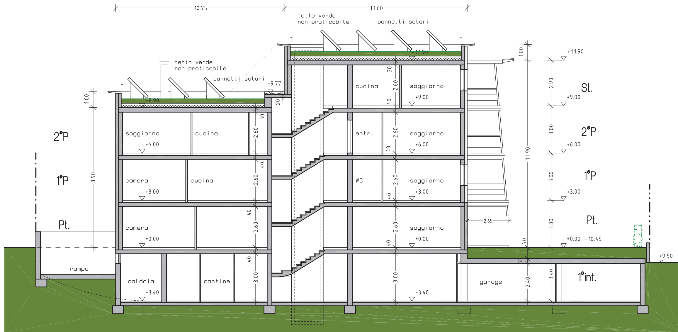
Schnitt B-B SEZIONE B-B
