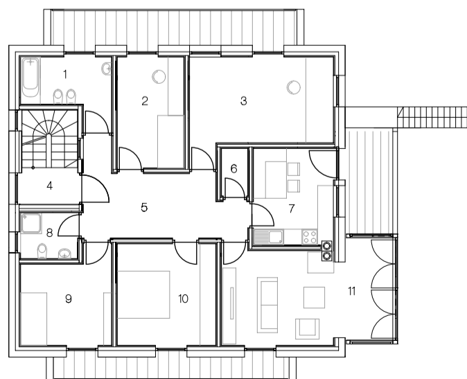
OBERGESCHOSS
