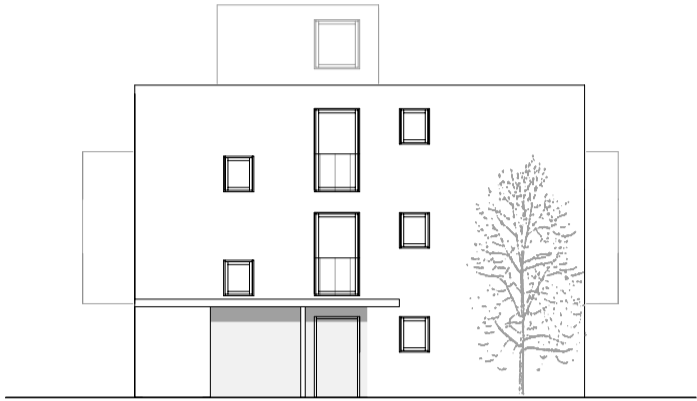
NORDANSICHT
