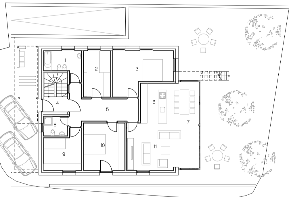
ERDGESCHOSS
