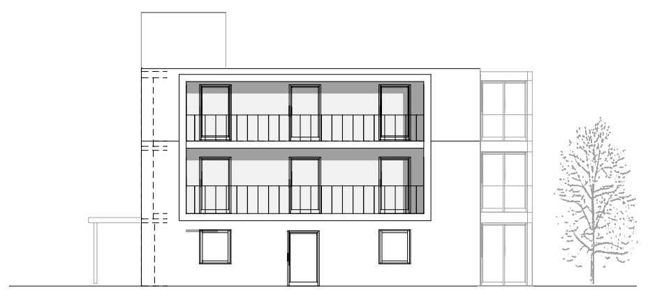
WESTANSICHT
