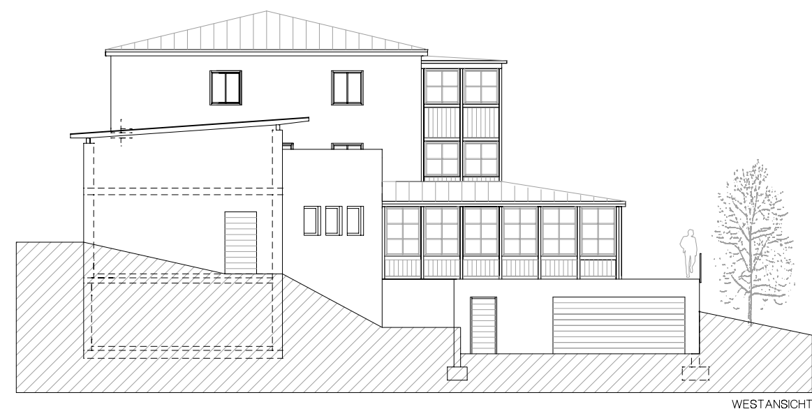
WESTANSICHT
