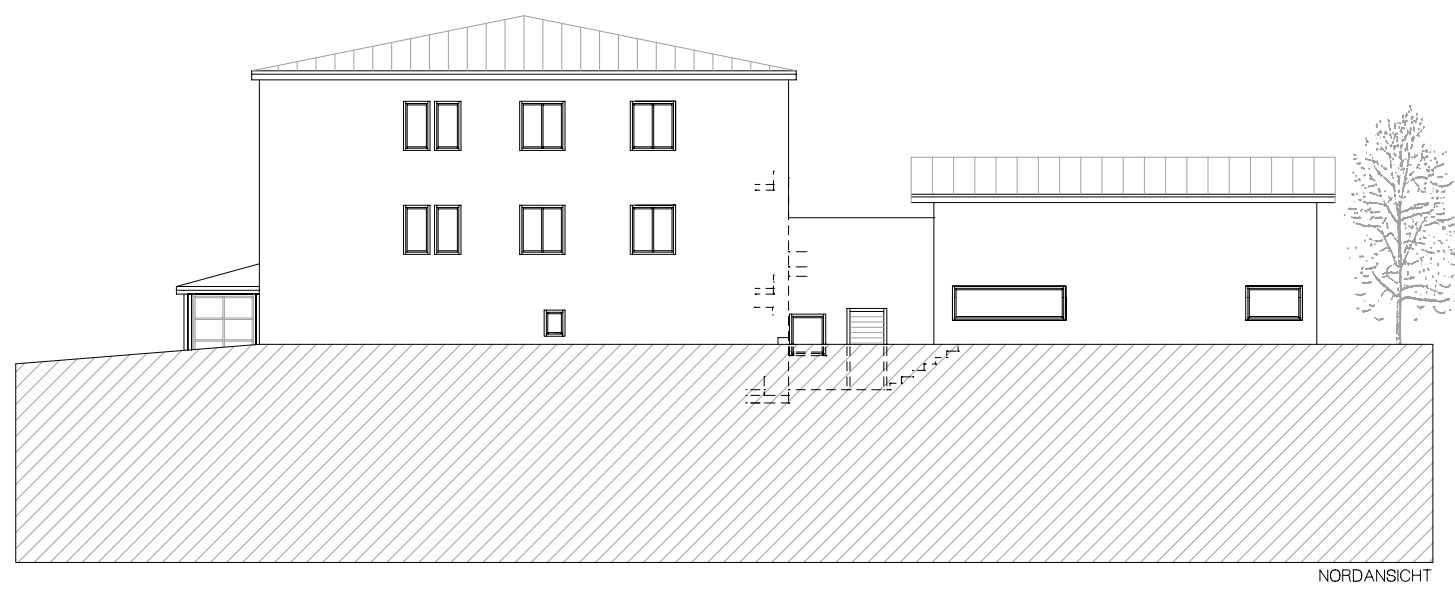
NORDANSICHT
