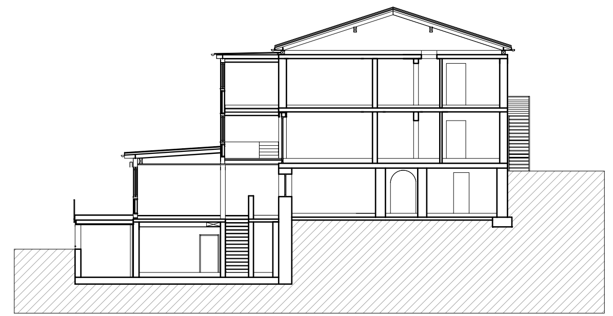
SCHNITT
