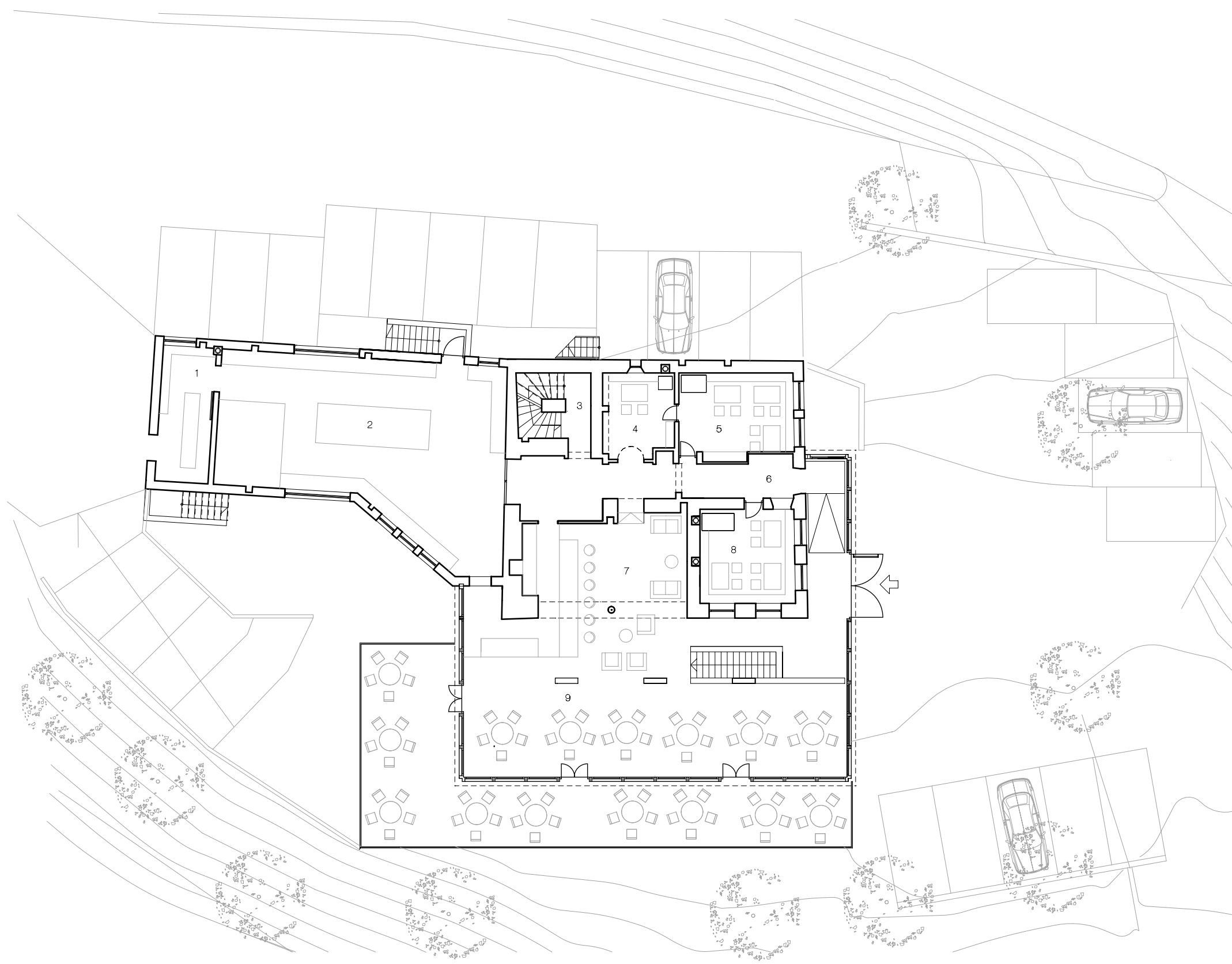
ERDGESCHOSS
