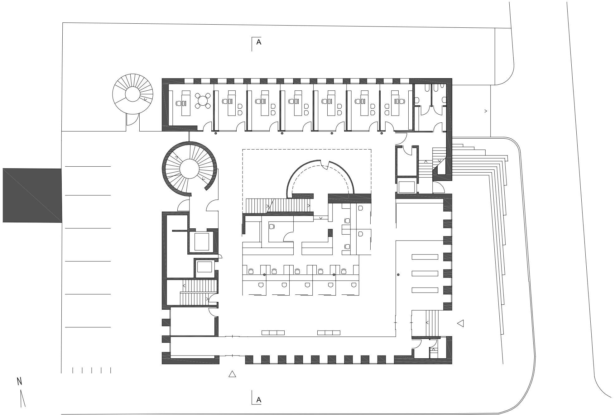
GRUNDRISS EBENE 0 - PIANTA LIVELLO 0
