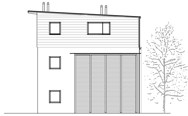
OSTANSICHT
