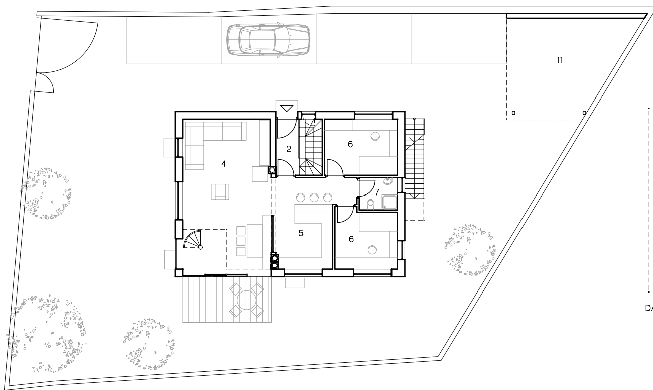
ERDGESCHOSS
