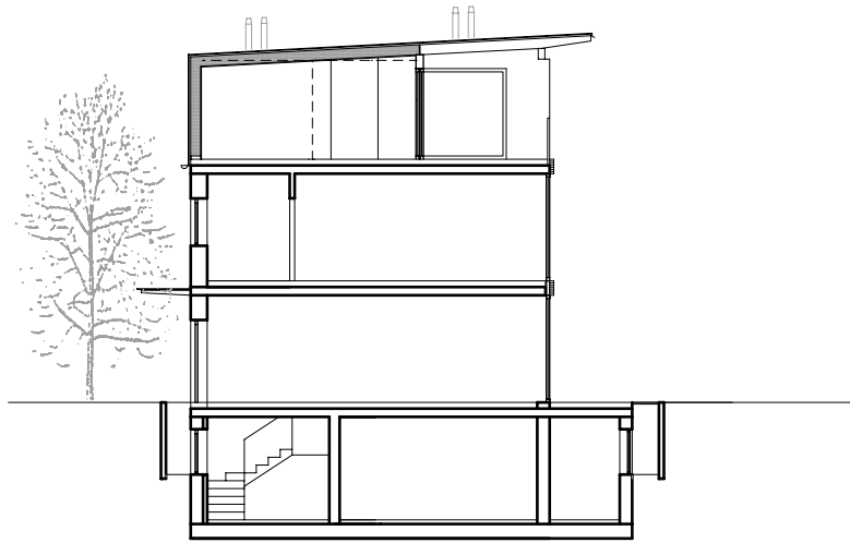
SCHNITT
