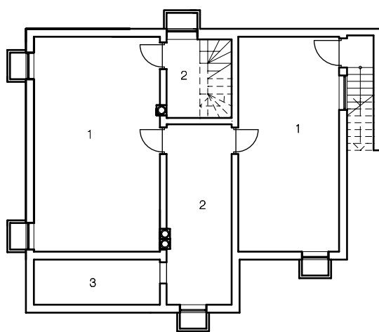
KELLERGESCHOSS
