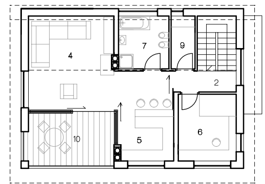
DACHGESCHOSS
