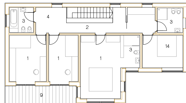
OBERGESCHOSS
