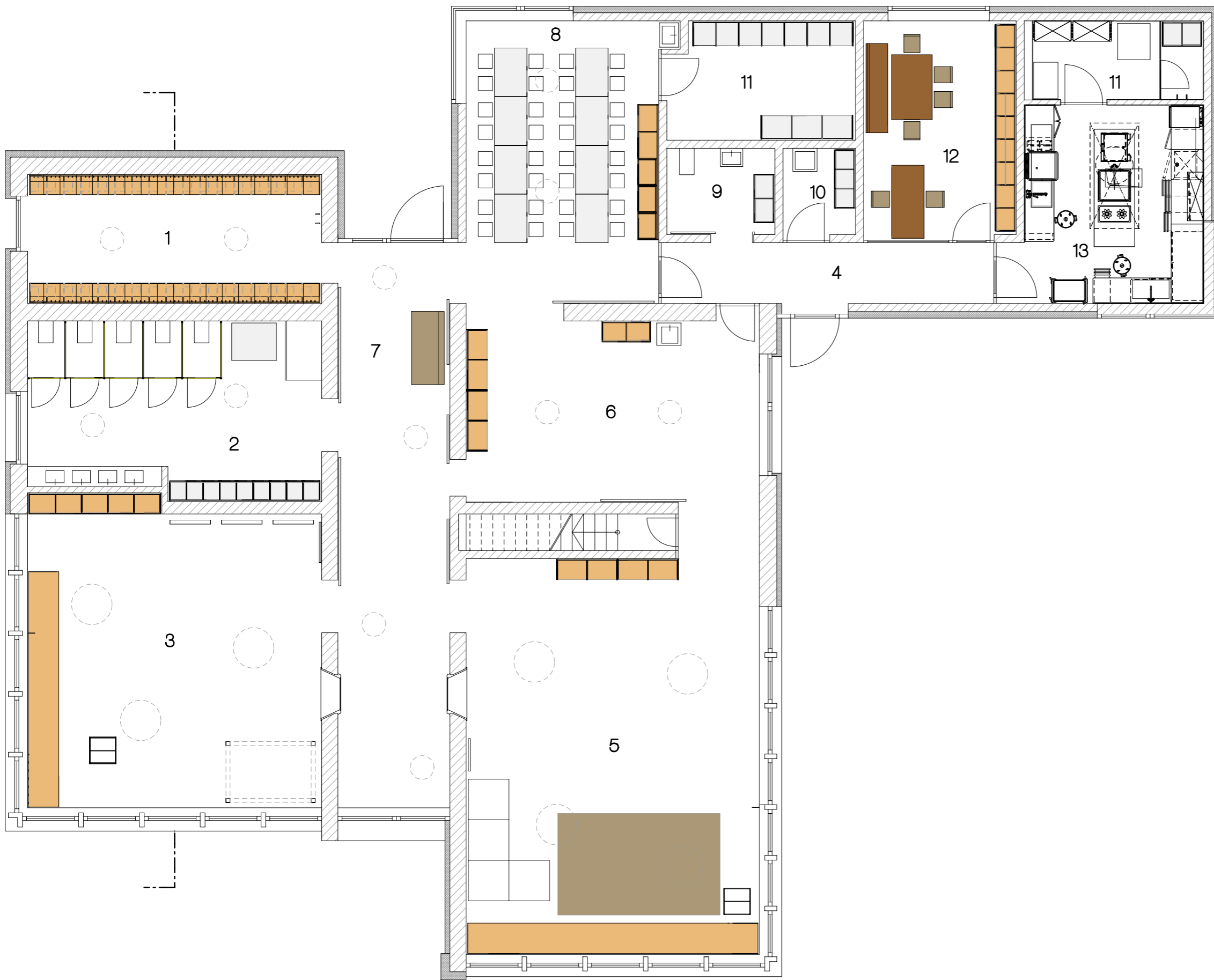
ERDGESCHOSS
