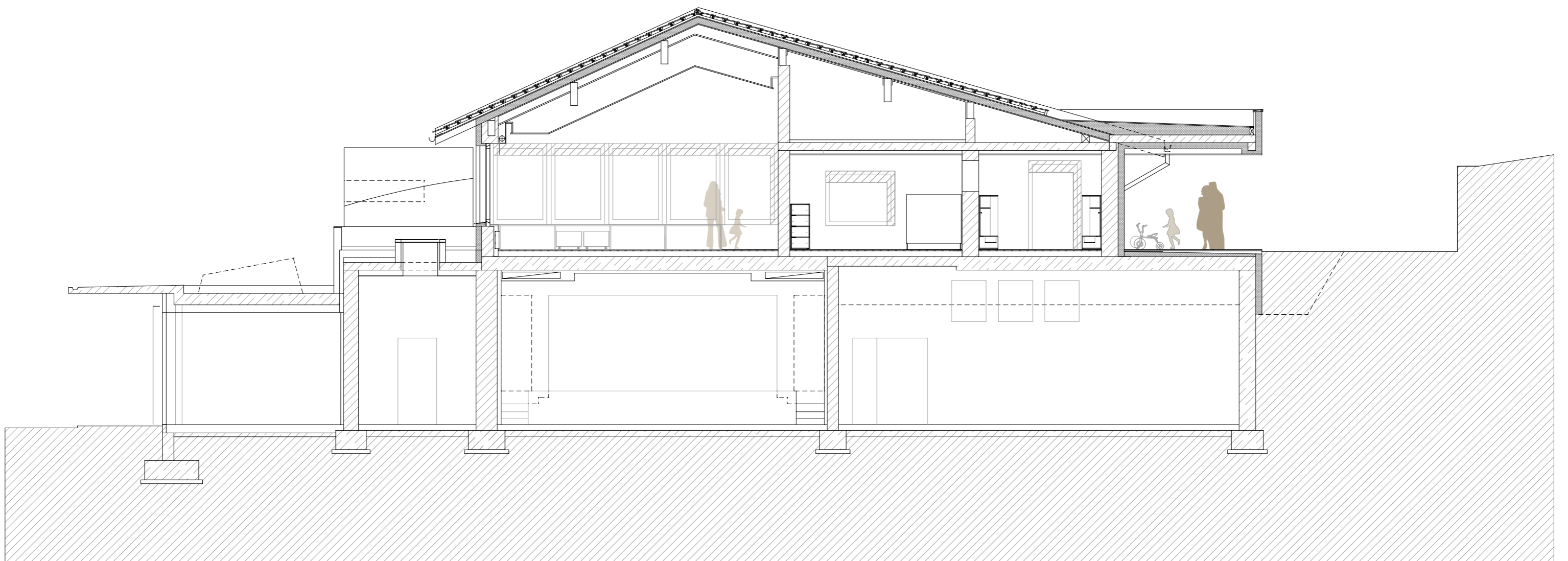
SCHNITT
