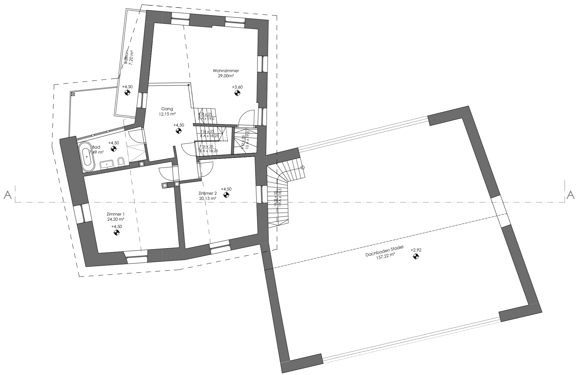
Obergeschoss - Endstand
