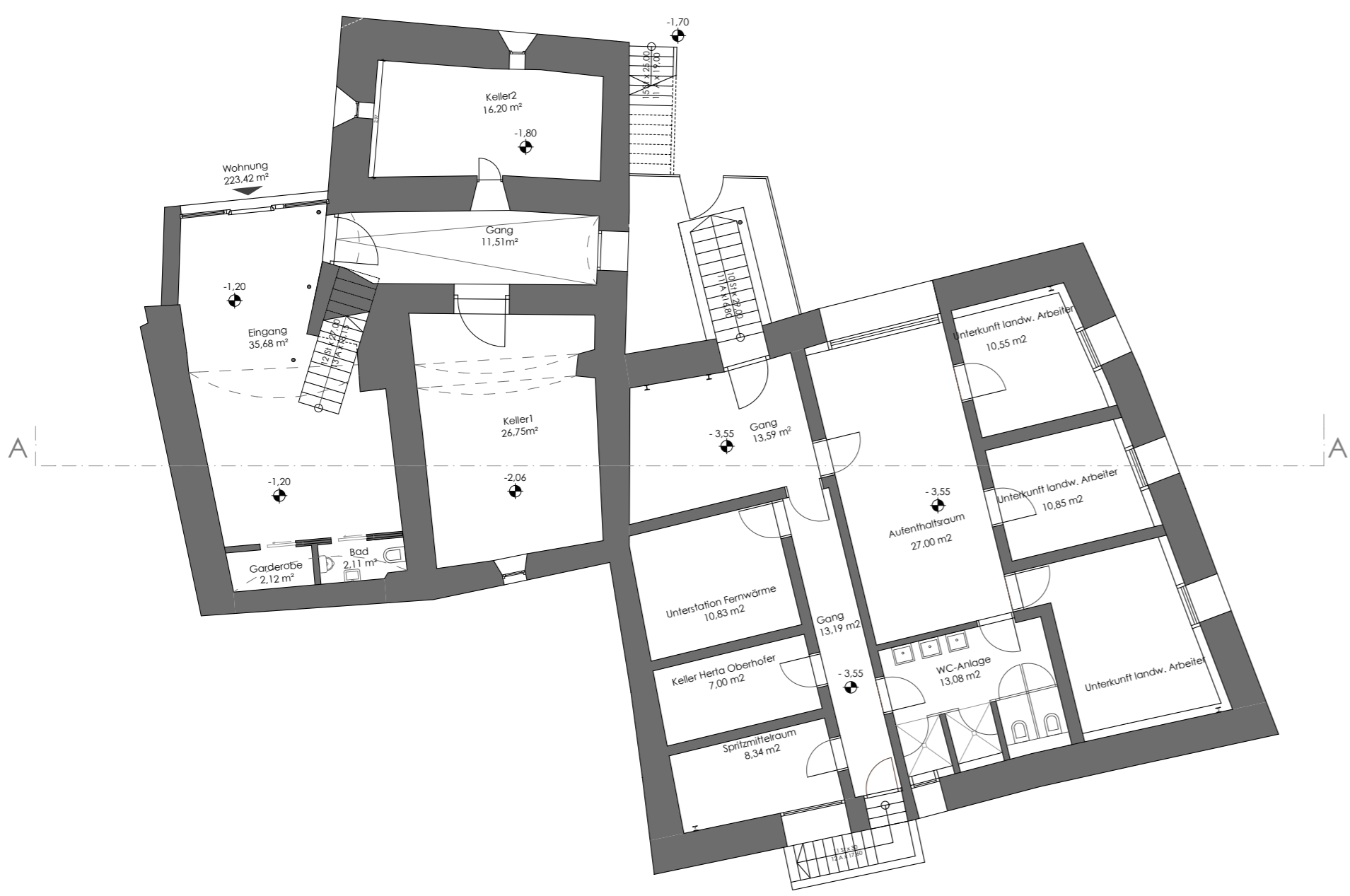
Kellergeschoss - Endstand
