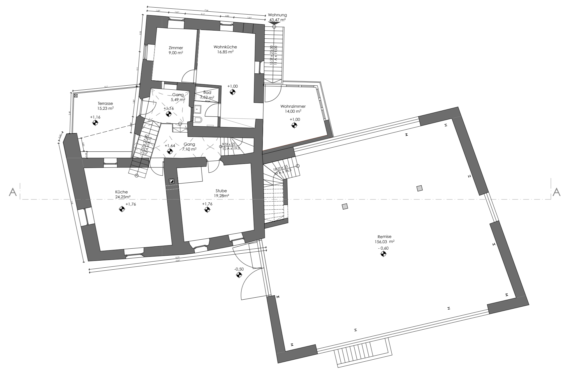
Erdgeschoss - Endstand
