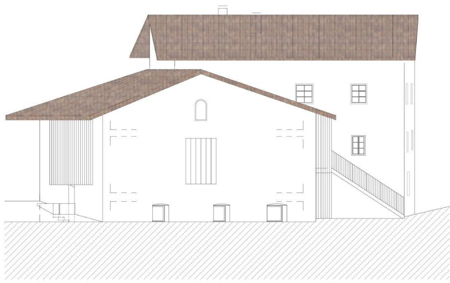
Nordansicht - Endstand
