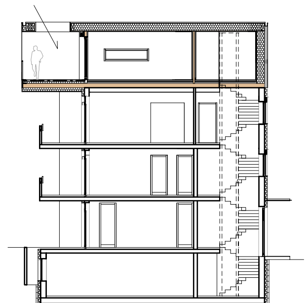
SCHNITT B-B
