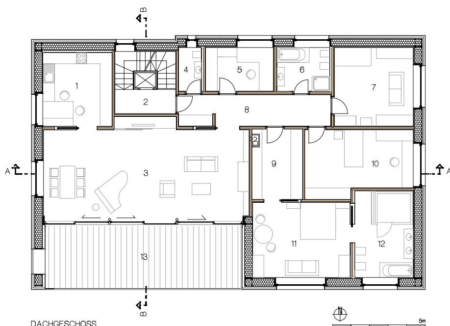
DACHGESCHOSS
