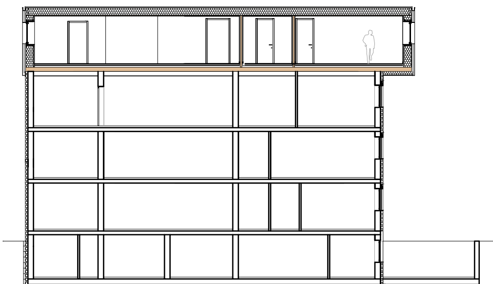
SCHNITT A-A
