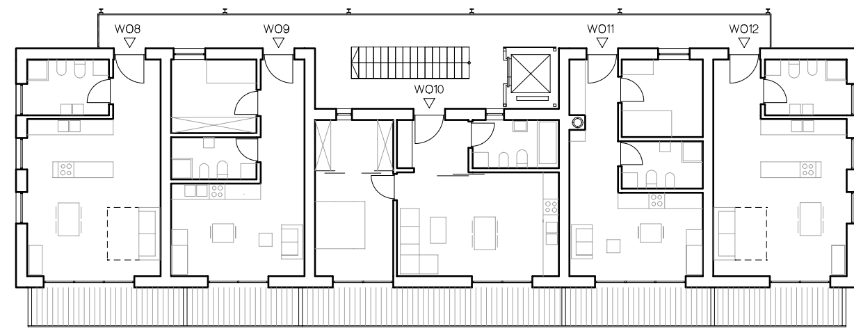
DACHGESCHOSS
