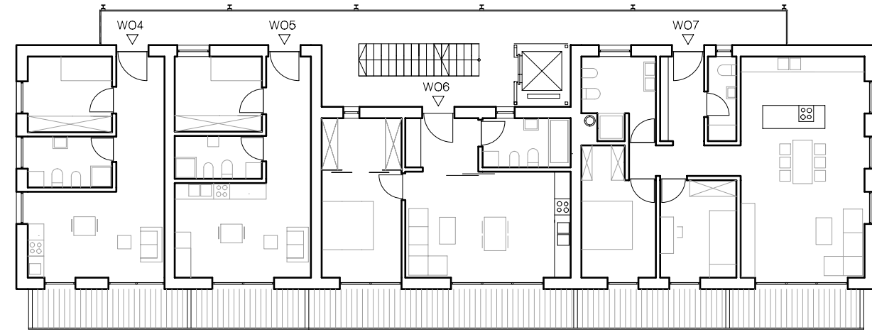
OBERGESCHOSS
