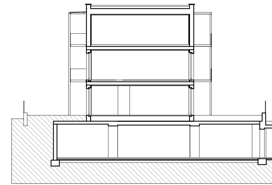
SCHNITT
