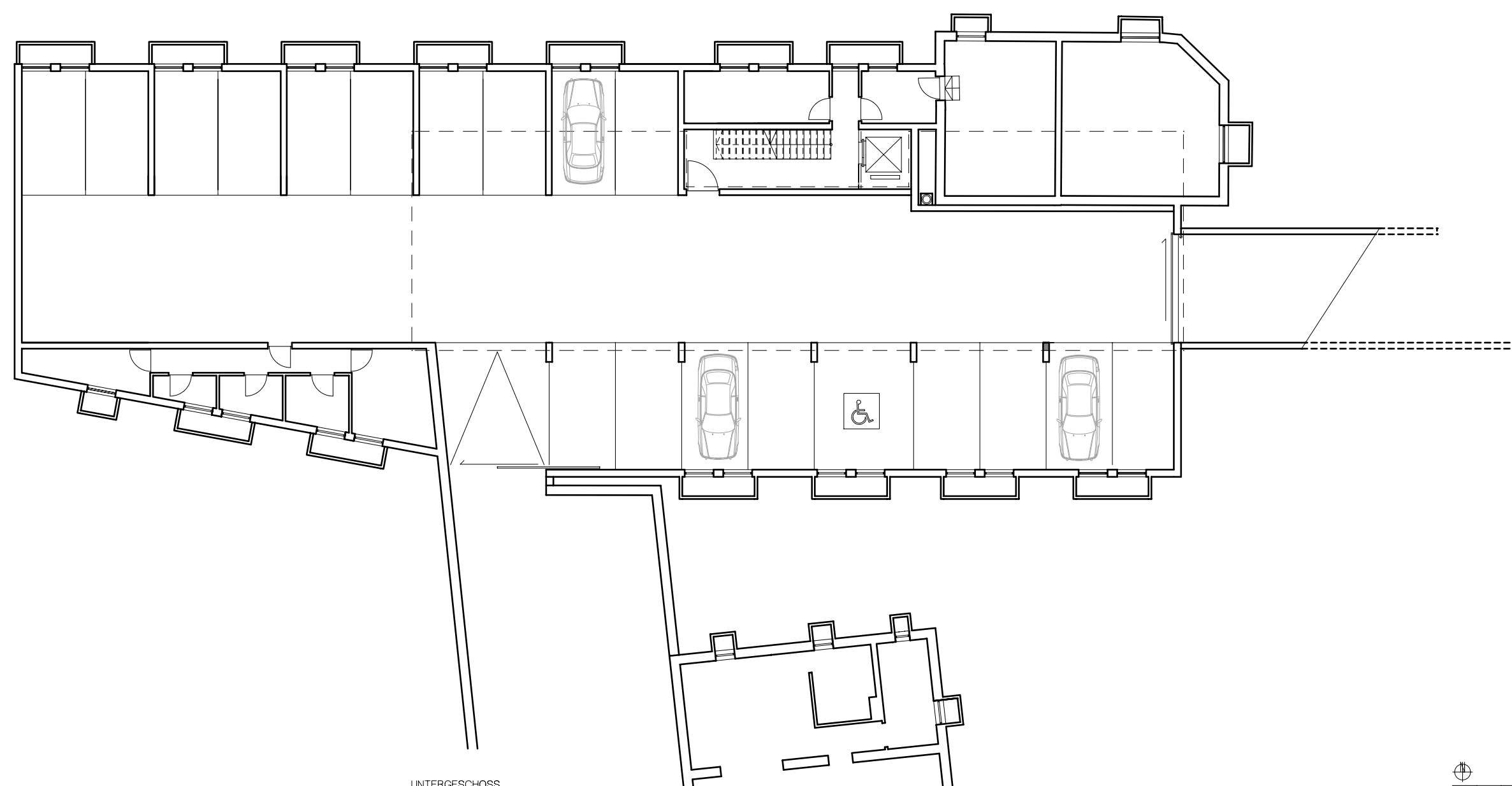
UNTERGESCHOSS
