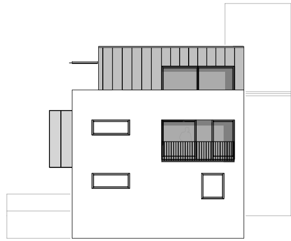
SÜDANSICHT
