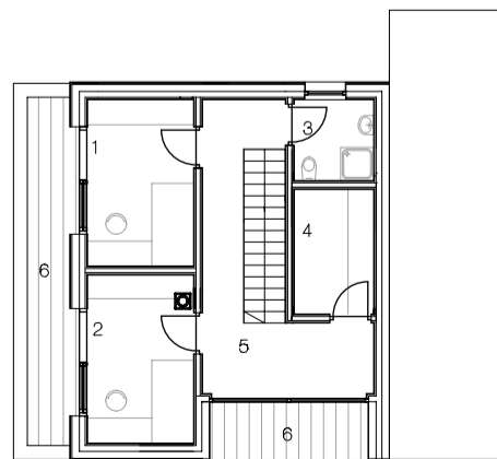
DACHGESCHOSS
