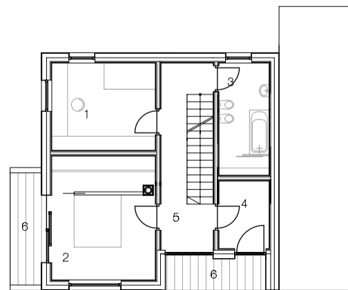
OBERGESCHOSS
