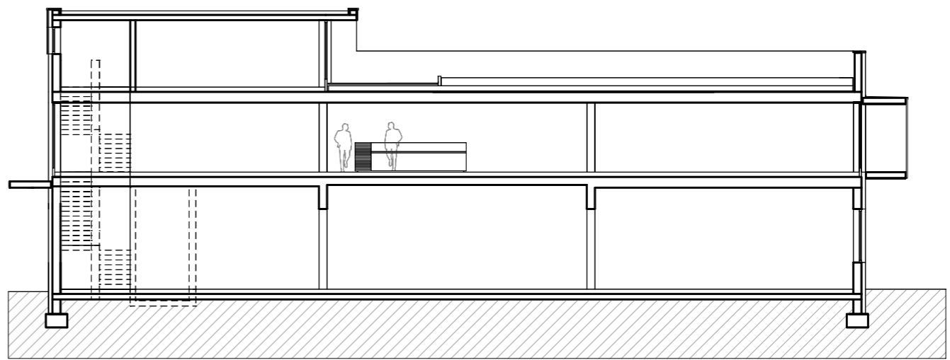
SCHNITT
