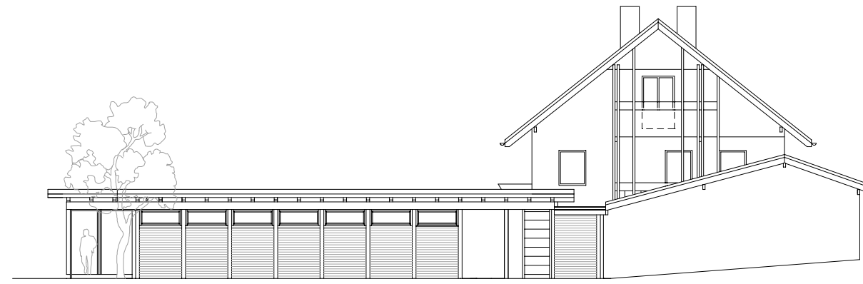
OSTANSICHT
