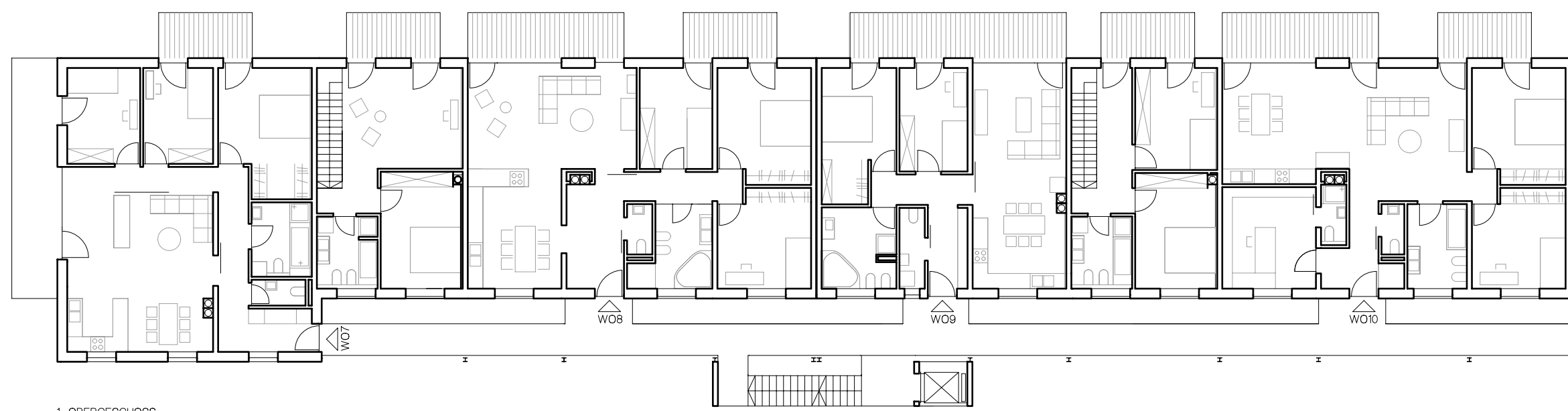
1. OBERGESCHOSS
