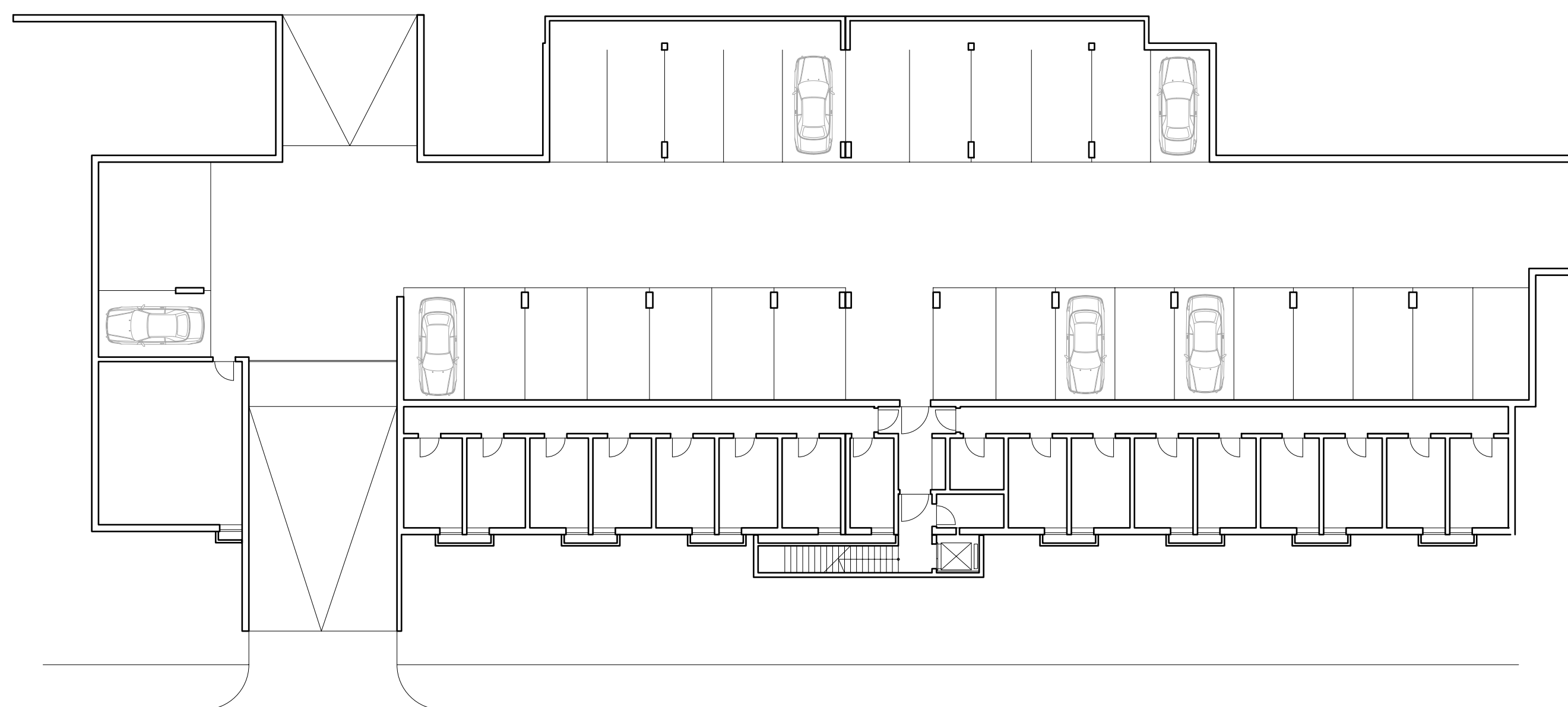
KELLERGESCHOSS
