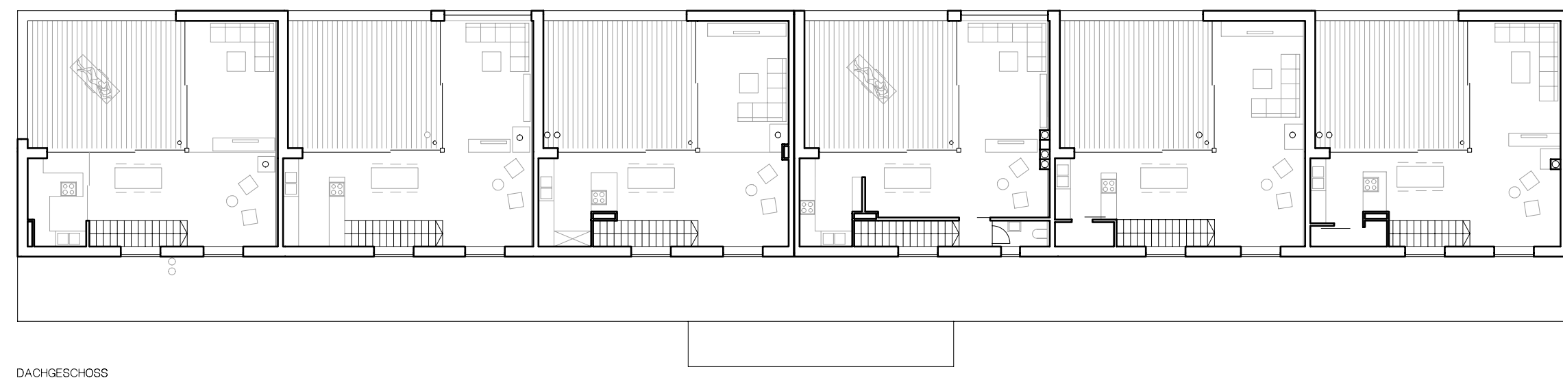
DACHGESCHOSS
