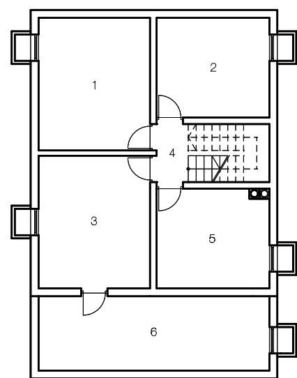
KELLERGESCHOSS
