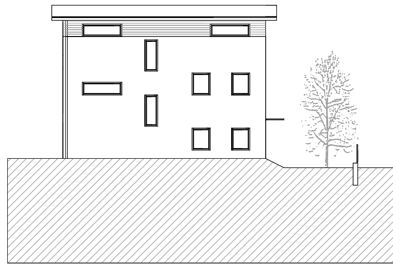
OSTANSICHT
