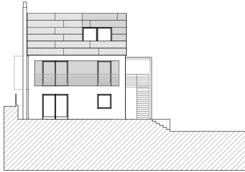
SUD ANSICHT
