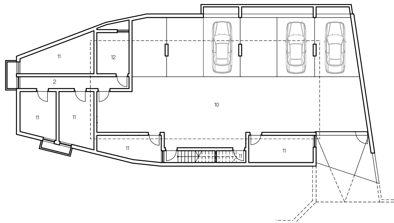
KELLERGESCHOSS
