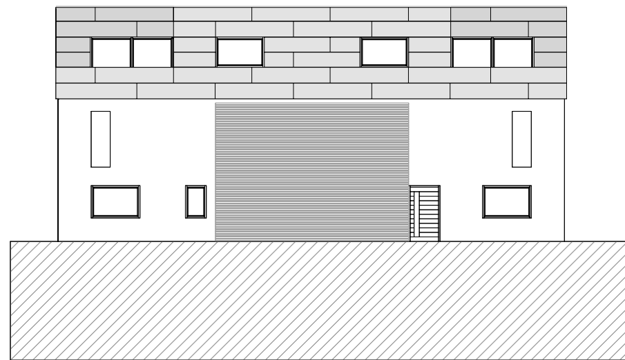
OST ANSICHT
