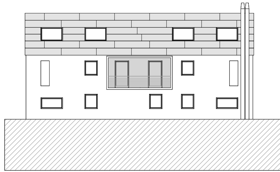
WEST ANSICHT
