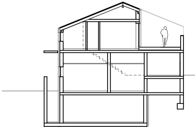
SCHNITT
