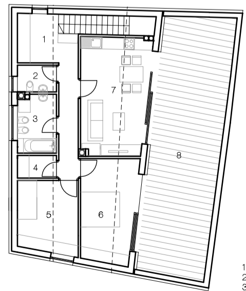
DACHGESCHOSS
