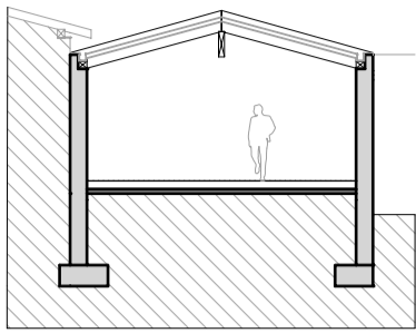
SCHNITT GERÄTERAUM
