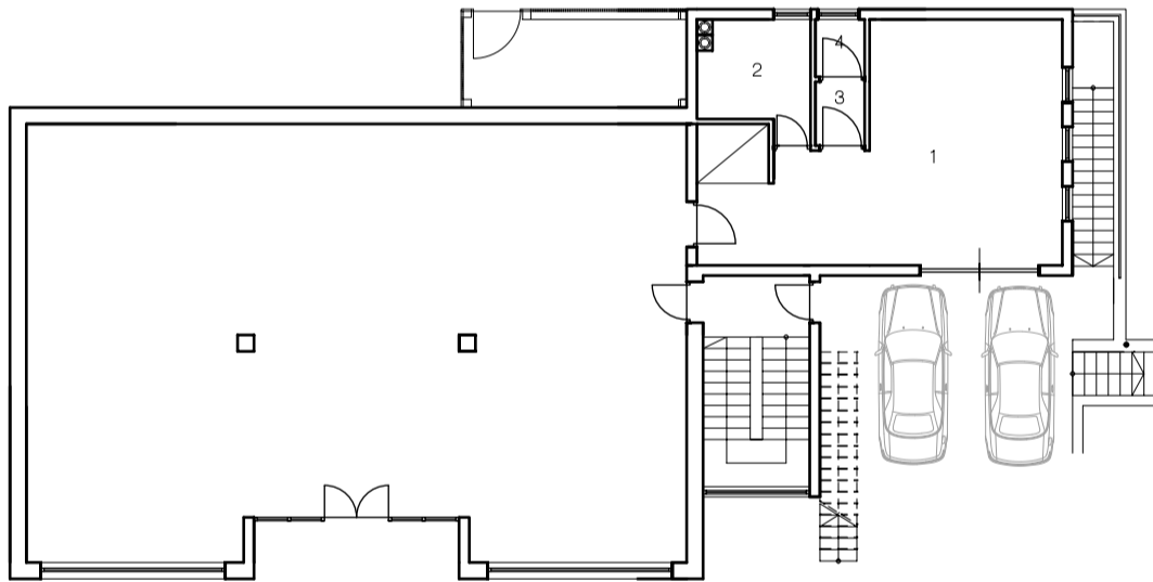
ERDGESCHOSS
