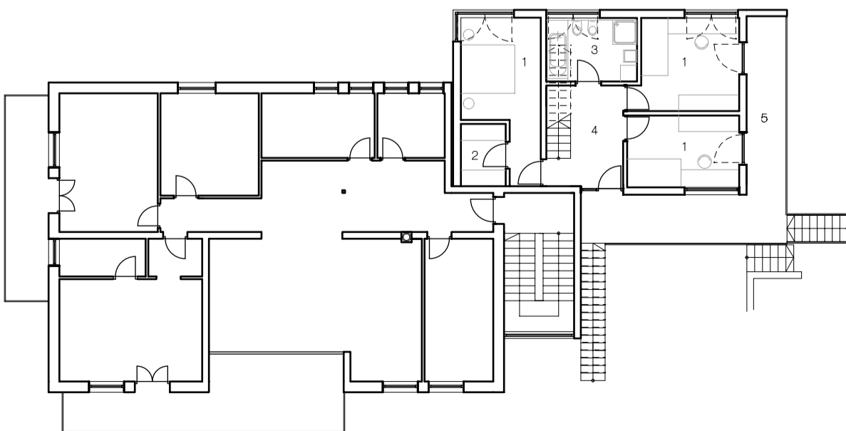
OBERGESCHOSS
