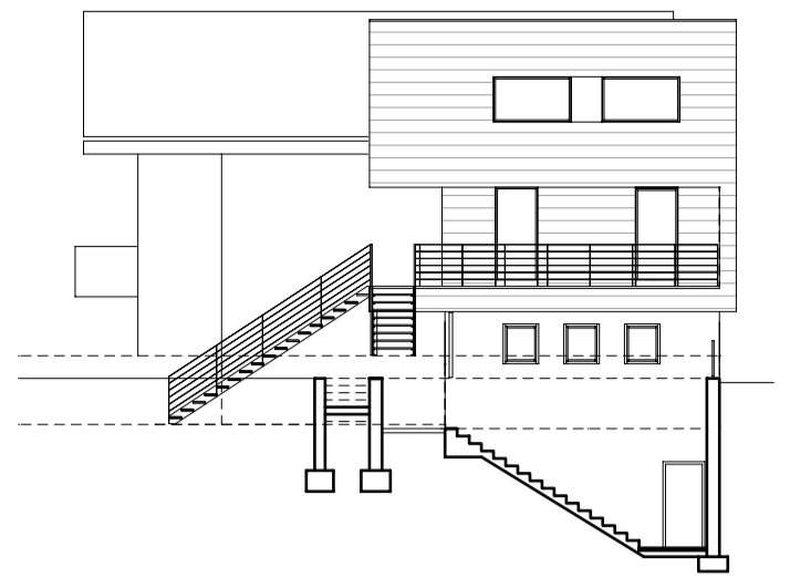
SÜD ANSICHT
