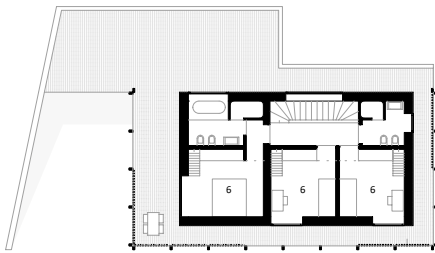
OBERGESCHOSS
