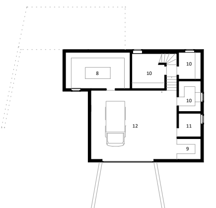
UNTERGESCHOSS
