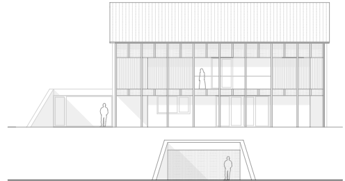
ANSICHT SÜD
