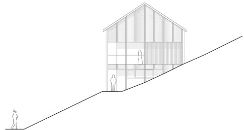
ANSICHT WEST
