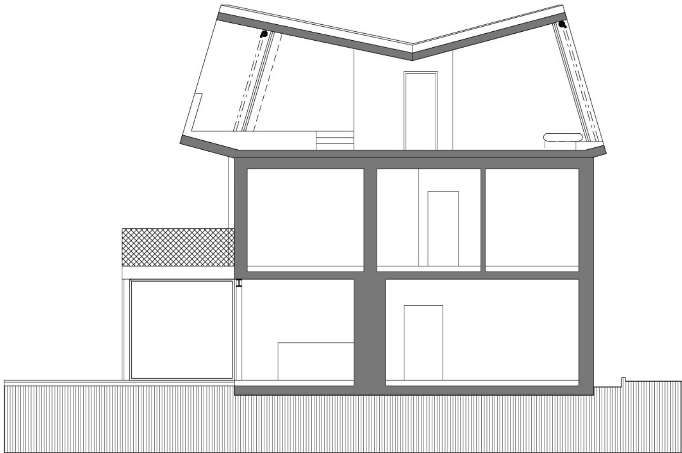
Schnitt A-A'
