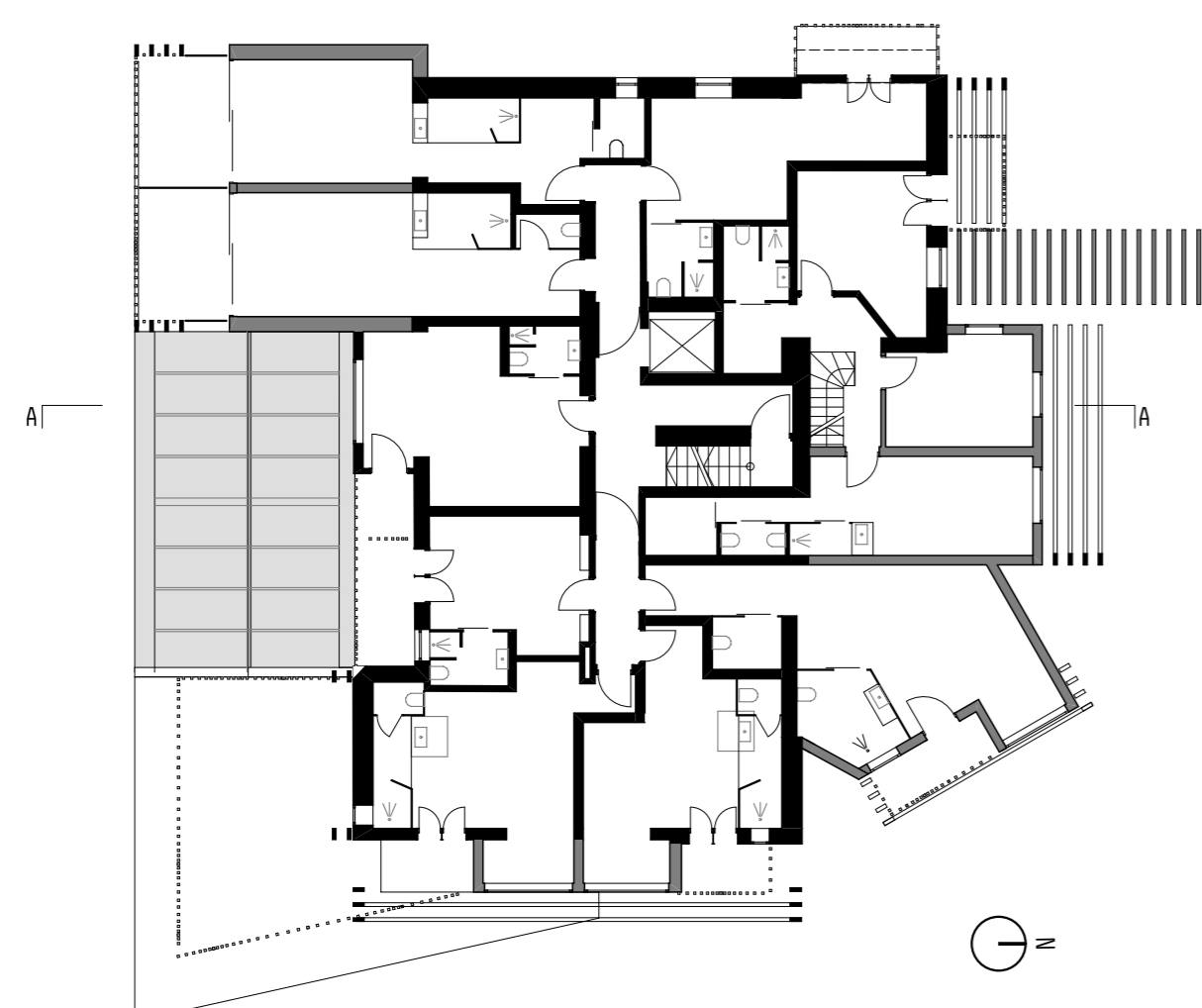
Grundriss OG 1 Plan first floor Pianta primo piano
