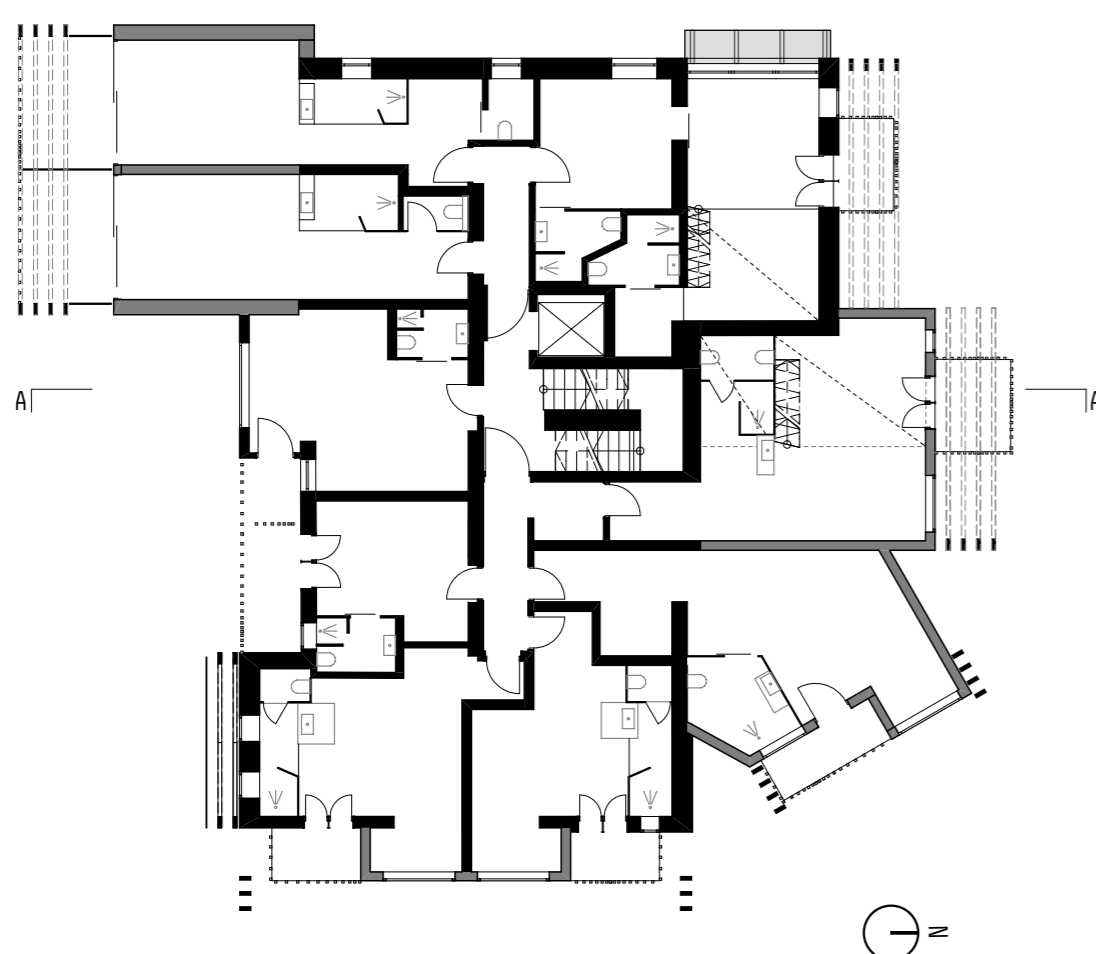
Grundriss OG 2 Plan second floor Pianta secondo piano
