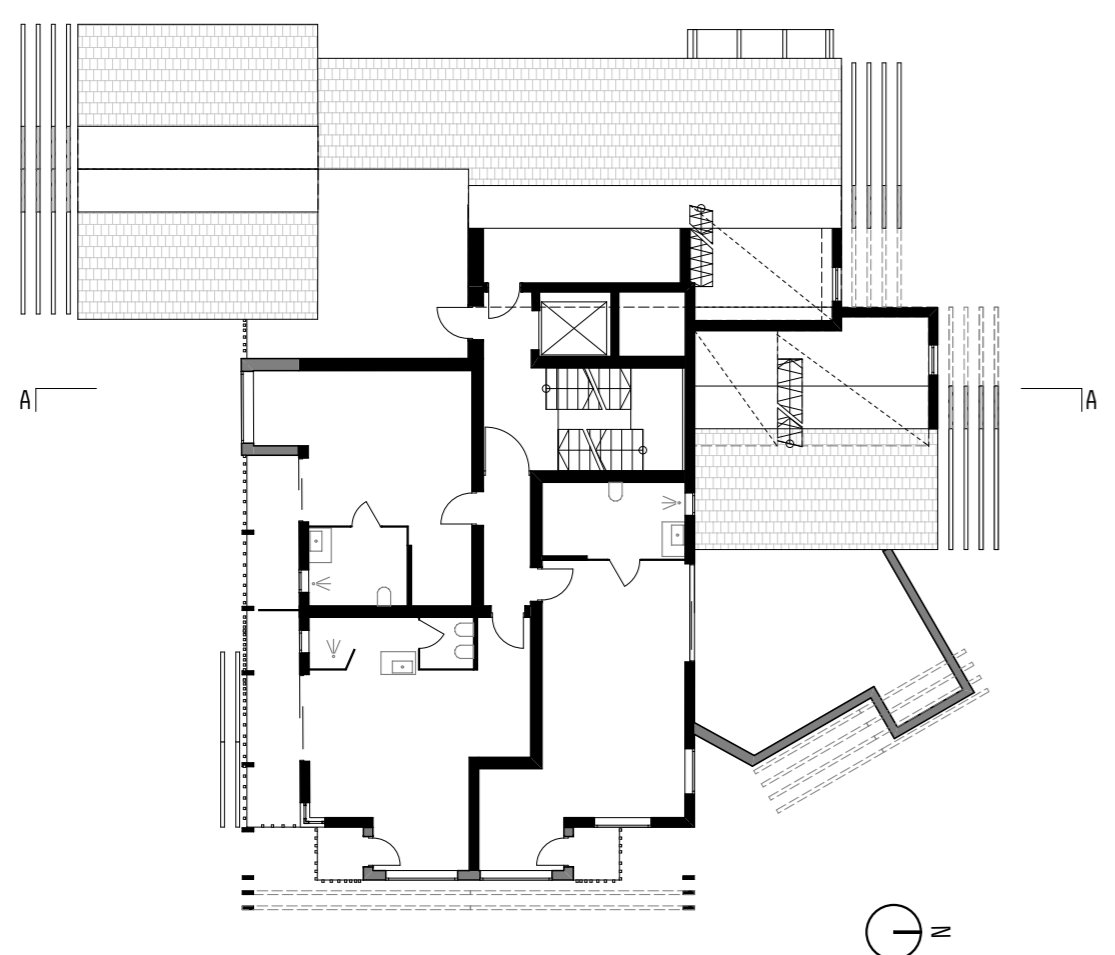
Grundriss OG 3 Plan third floor Pianta terzo piano
