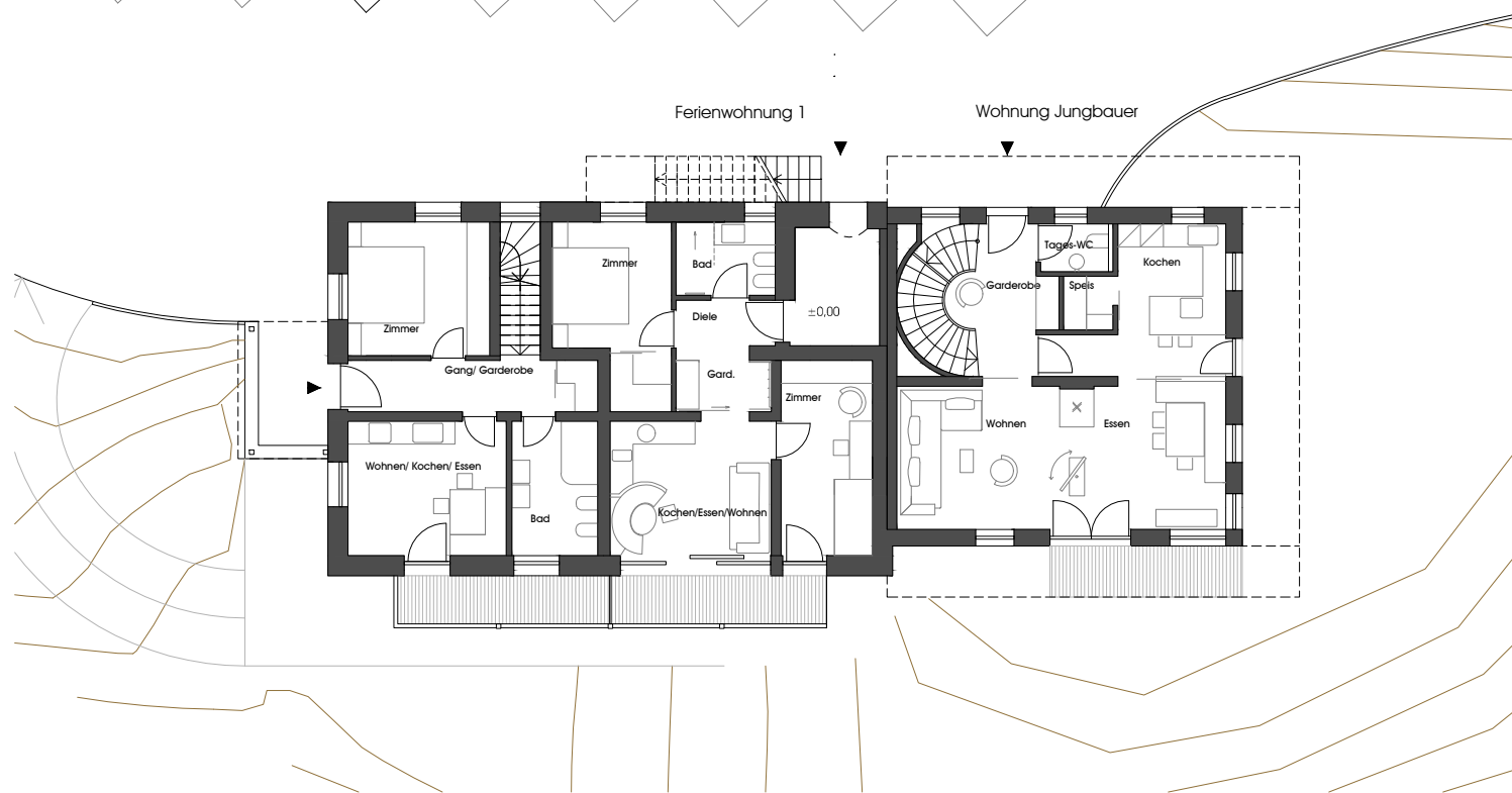
ERDGESCHOSS
