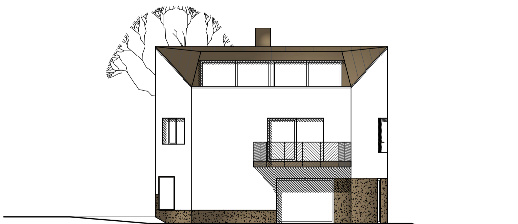
WESTANSICHT
