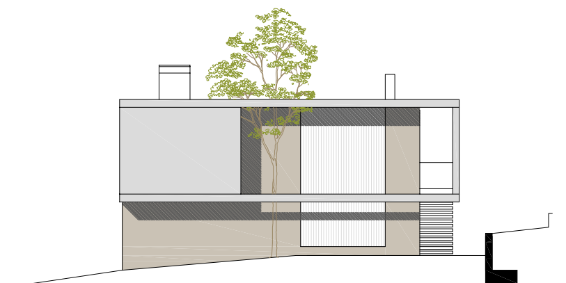
NORD PROSPECT
