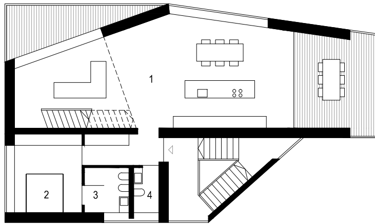
OBERGESCHOSS
