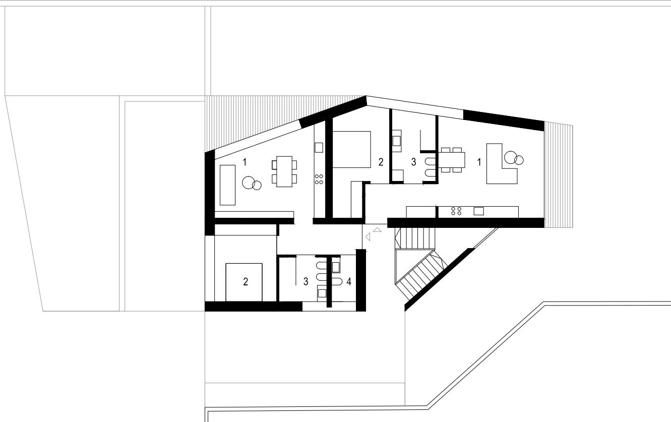
ERDGESCHOSS
