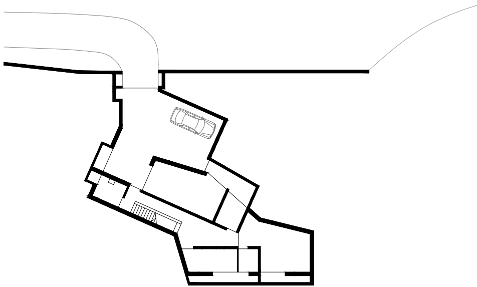
KELLERGESCHOSS
