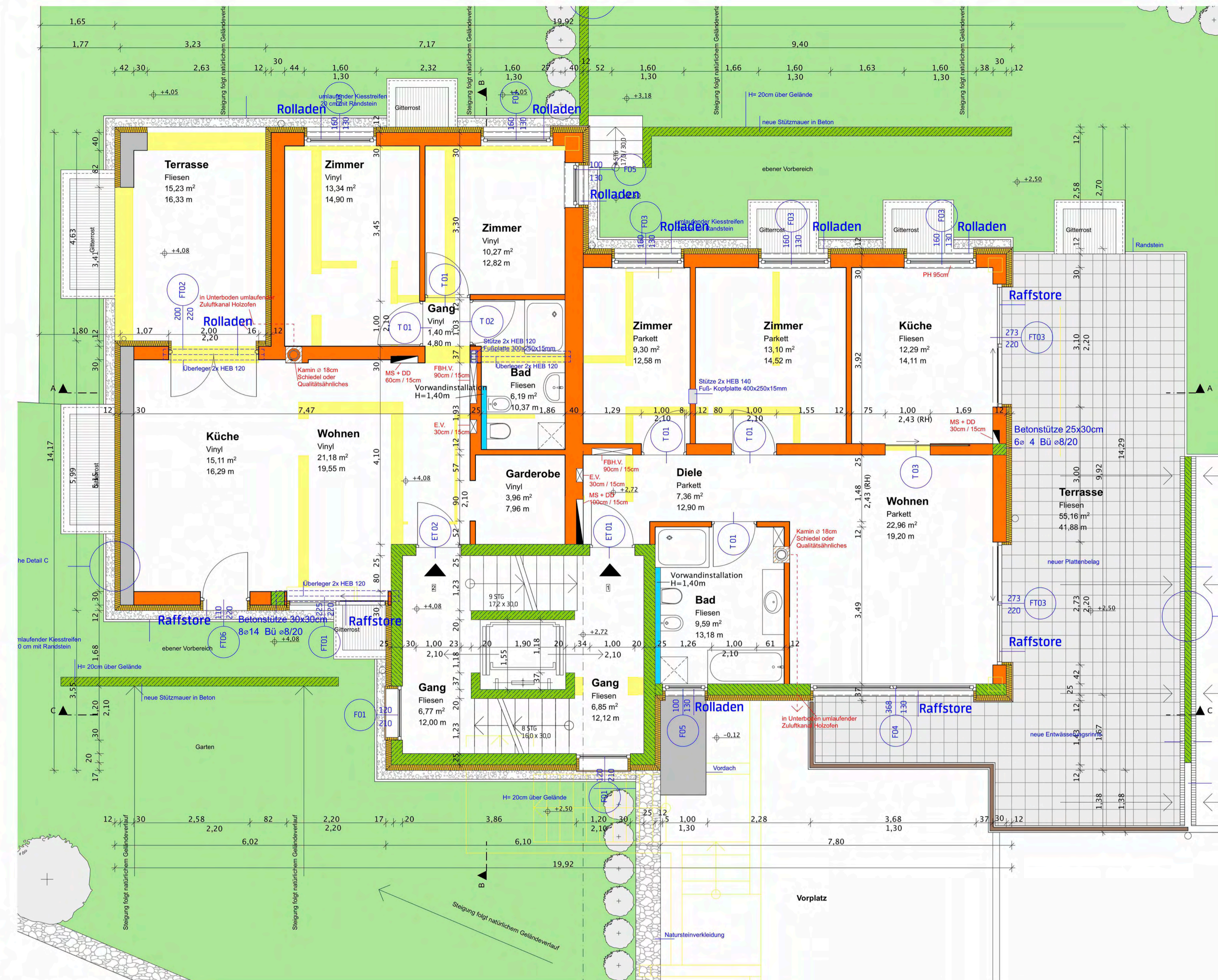
ERDGESCHOSS
