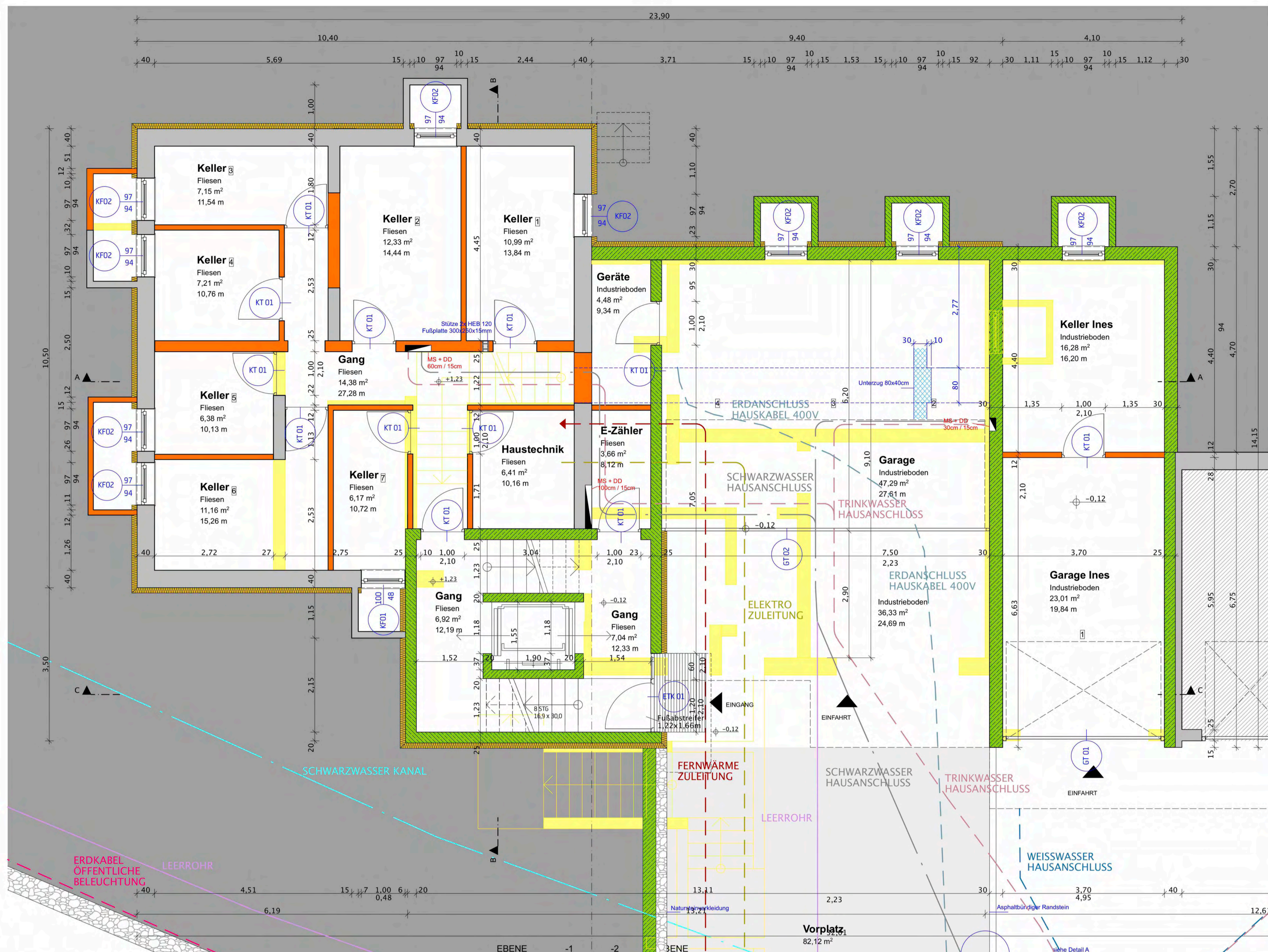
KELLERGESCHOSS
