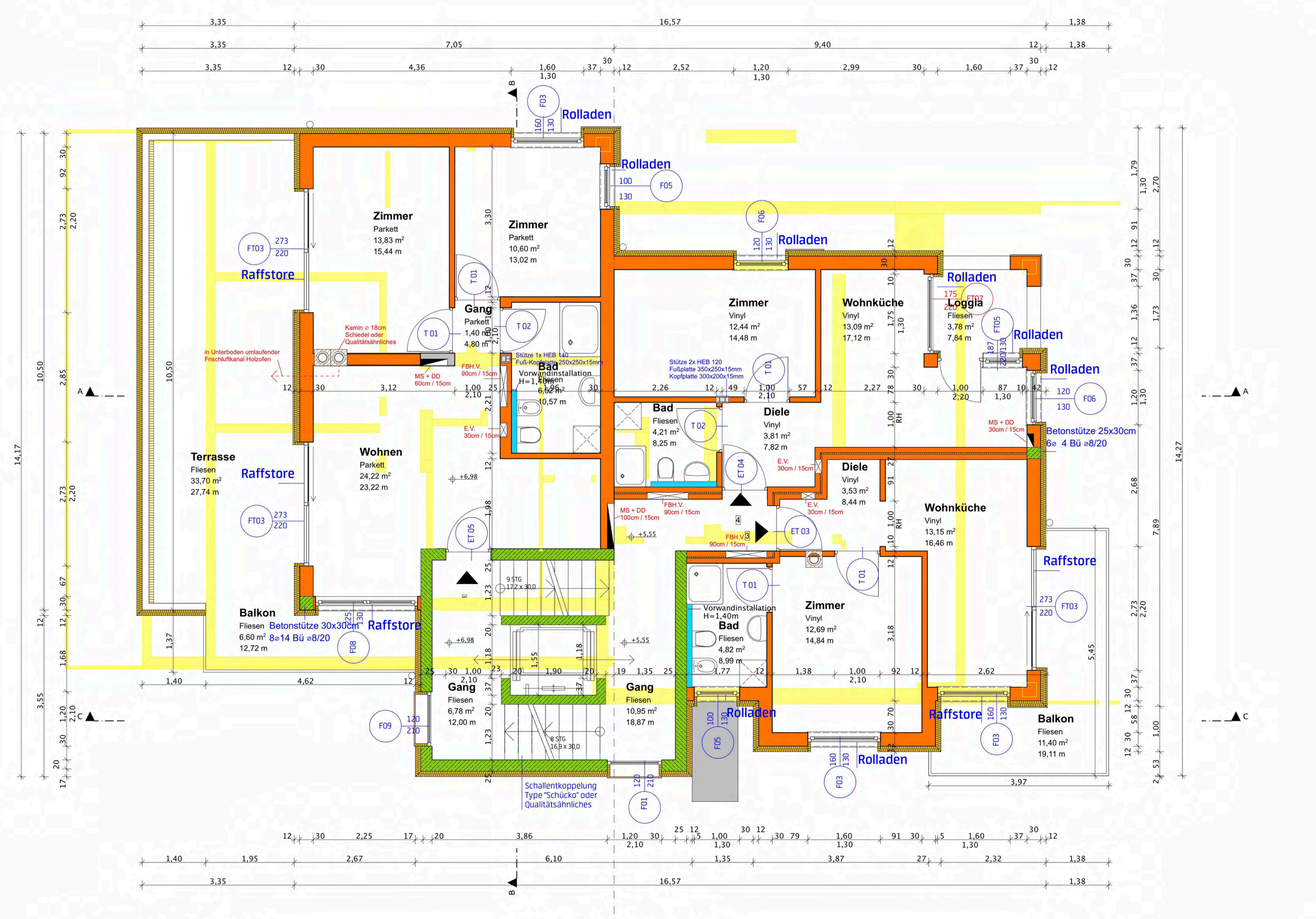
1. OBERGESCHOSS
