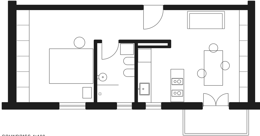
GRUNDRISS 1:100
