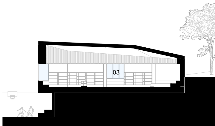
SEZIONE A-A
