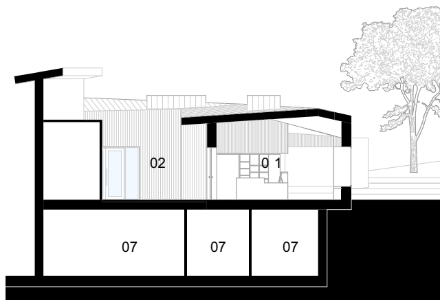
SEZIONE C-C
