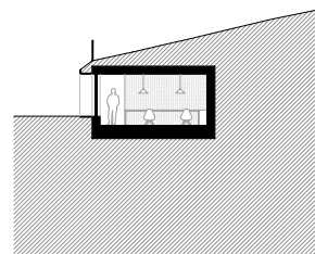
SCHNITT
