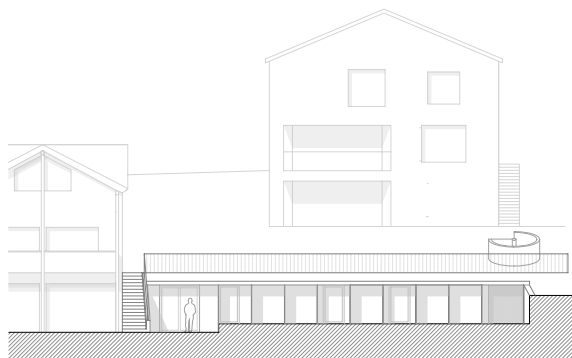
ANSICHT SÜD
