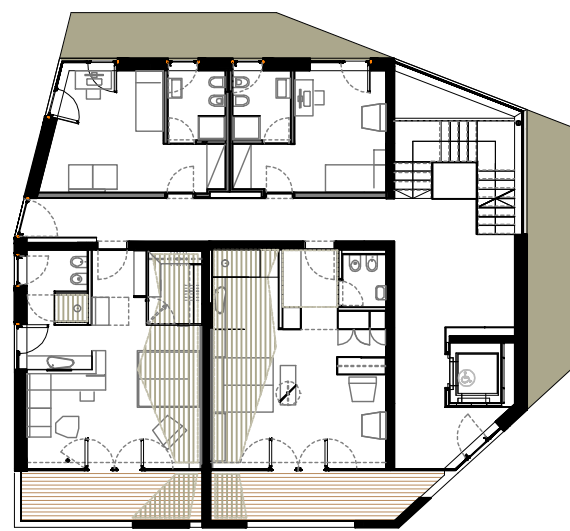
ERSTE GESCHOSSEBENE
