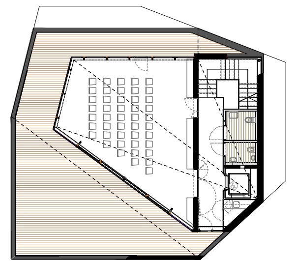
DACHTERRASSENEBENE
