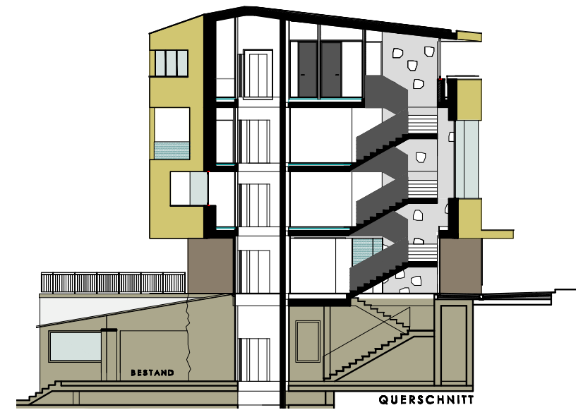
QUERSCHNITT
