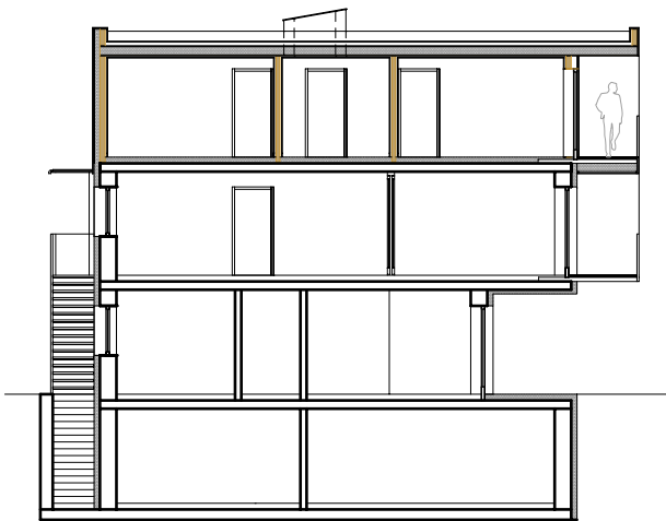
SCHNITT
