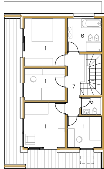
DACHGESCHOSS
