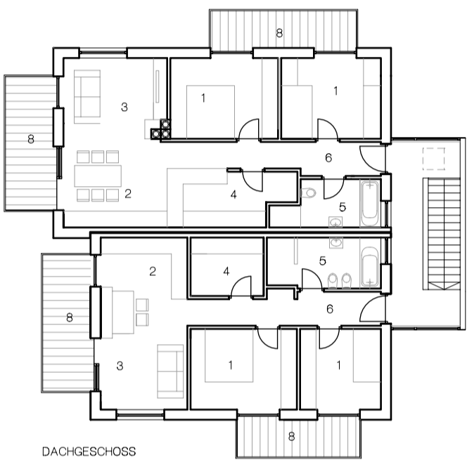
DACHGESCHOSS
