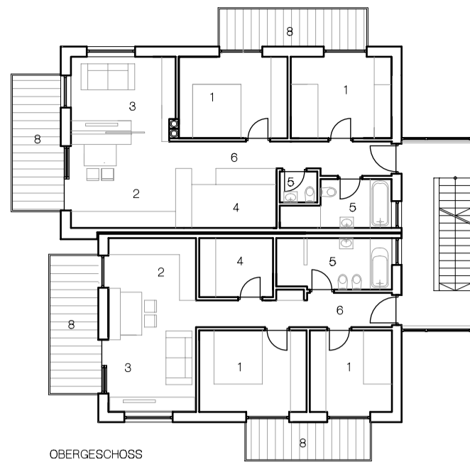
OBERGESCHOSS
