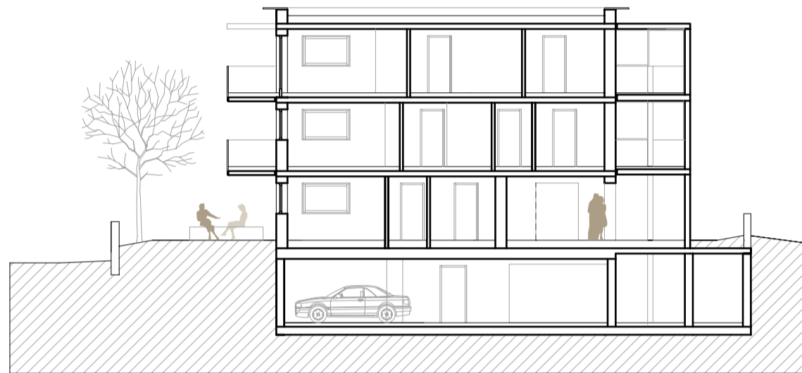
SCHNITT AA
