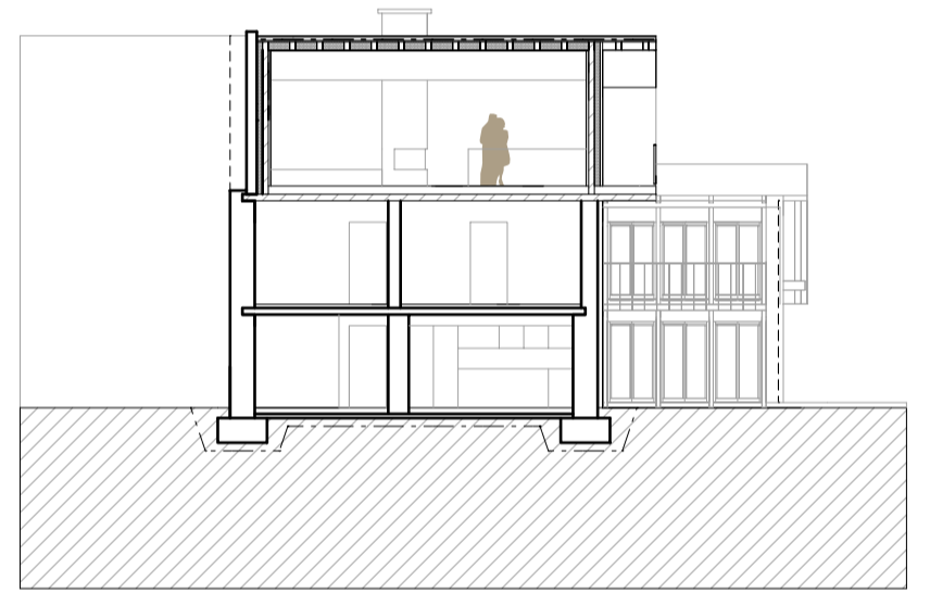
SCHNITT BB
