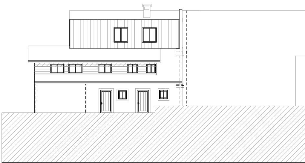
NORDANSICHT
