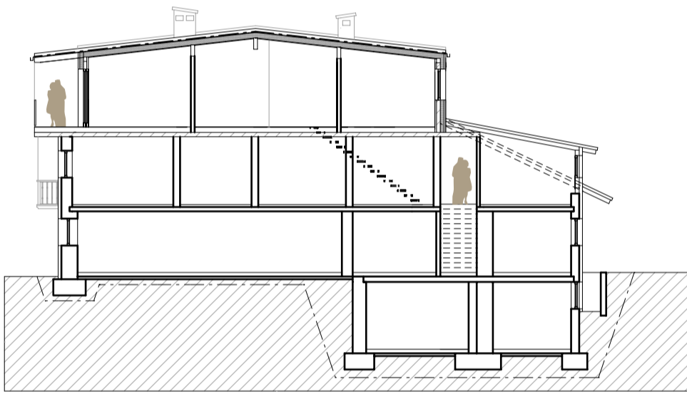
SCHNITT AA
