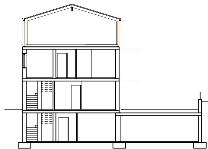
SCHNITT
