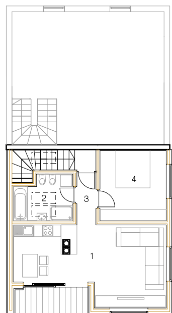
DACHGESCHOSS
