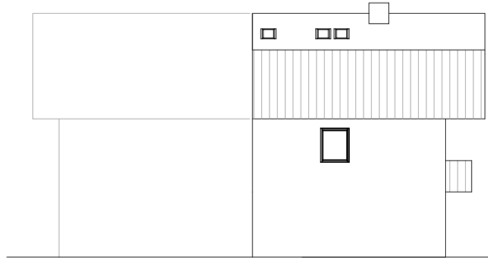
WESTANSICHT
