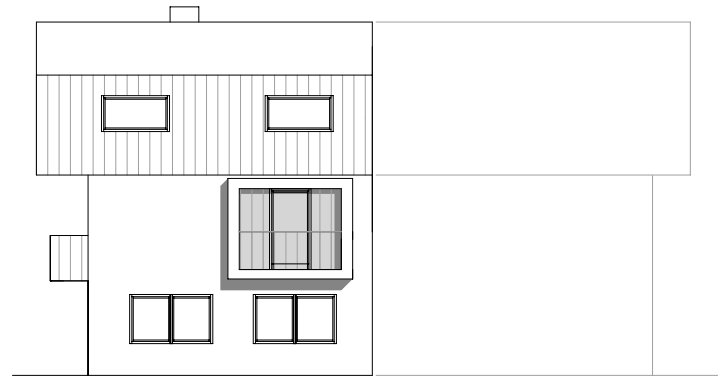
OSTANSICHT
