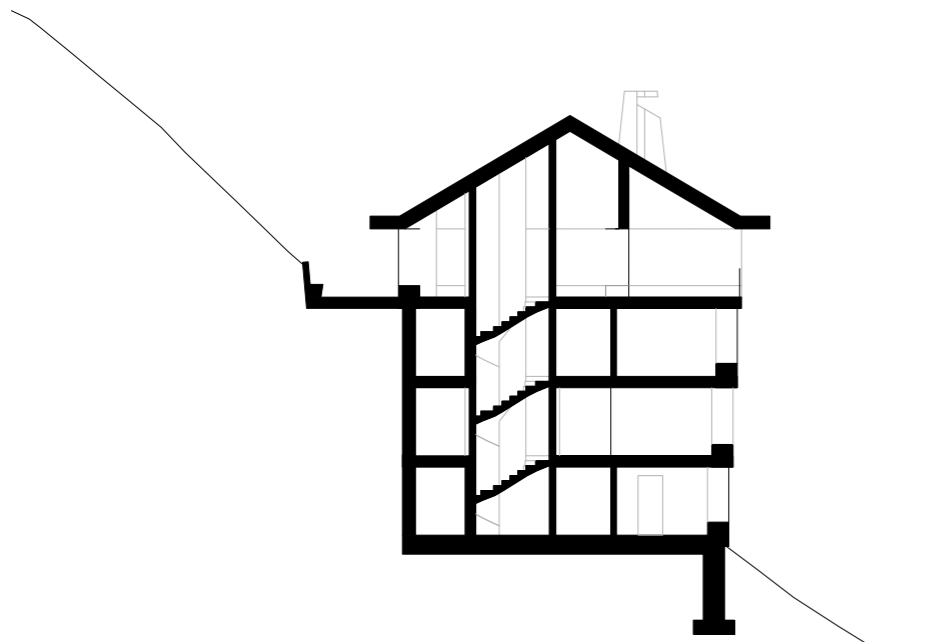
QUERSCHNITT
