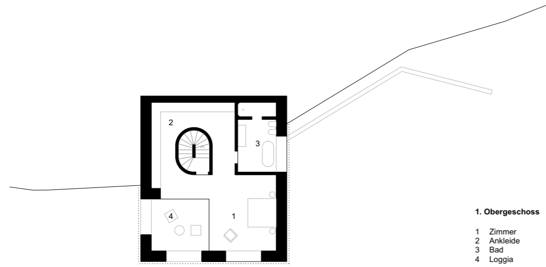
1. OBERGESCHOSS
