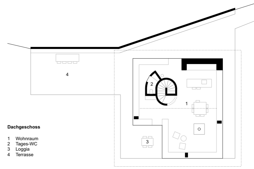
DACHGESCHOSS
