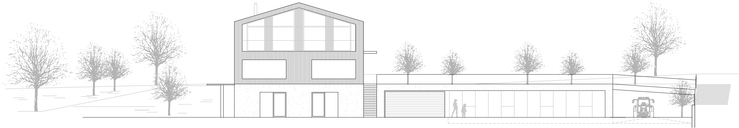
ANSICHT OST
