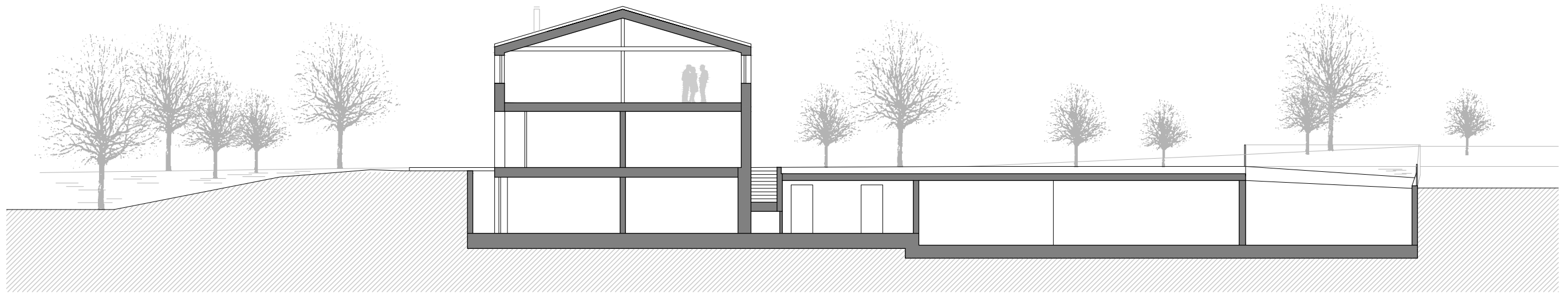
SCHNITT
