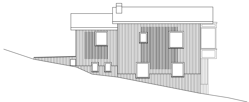
Ost Ansicht - prospetto ovest
