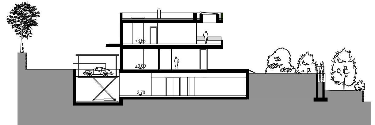
HOUSE M_SECTION A:A
