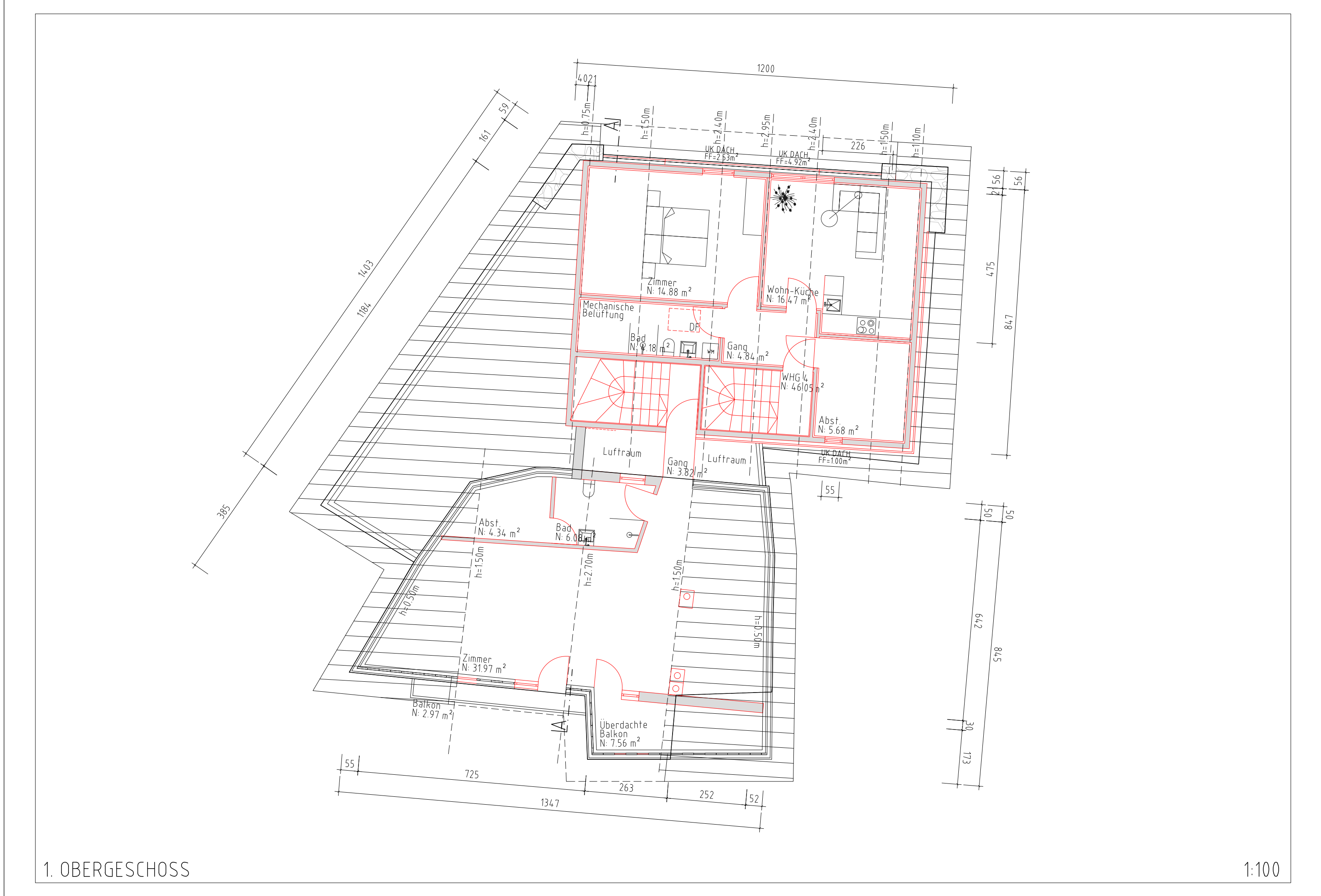
1. OBERGESCHOSS
