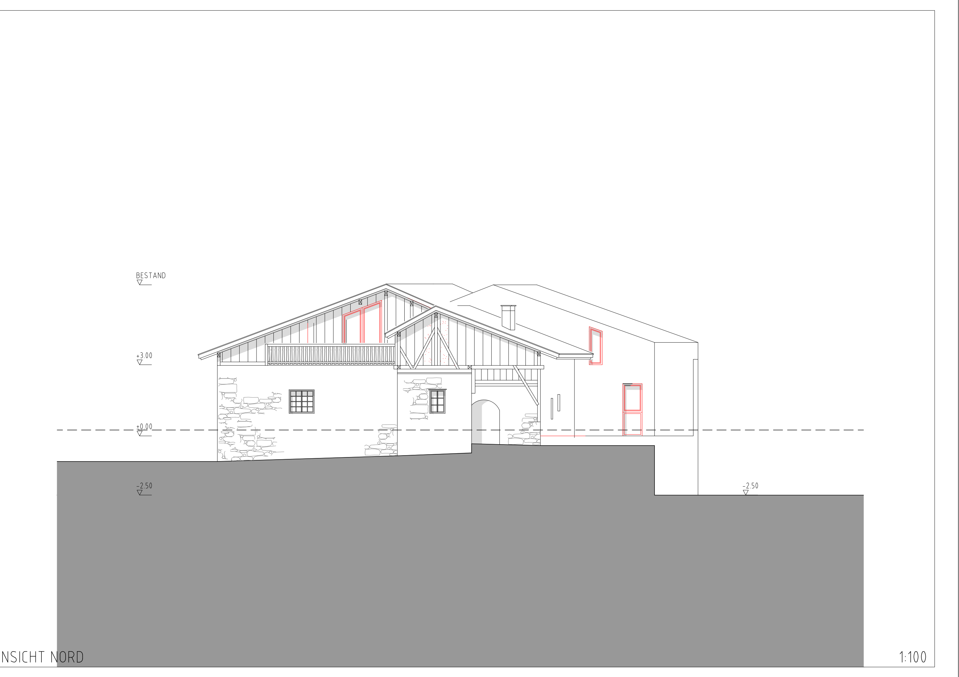
ANSICHT NORD
