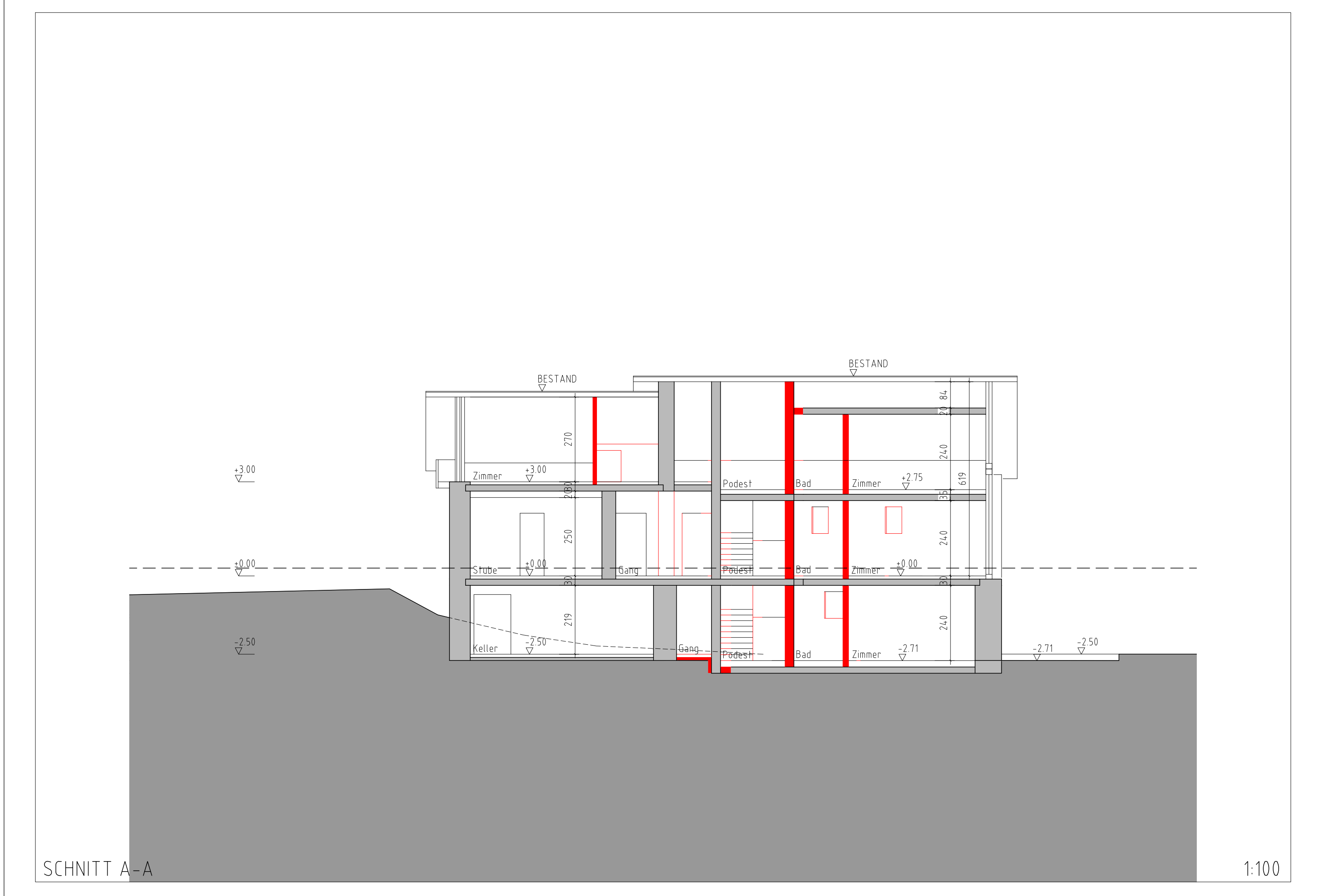
SCHNITT A-A
