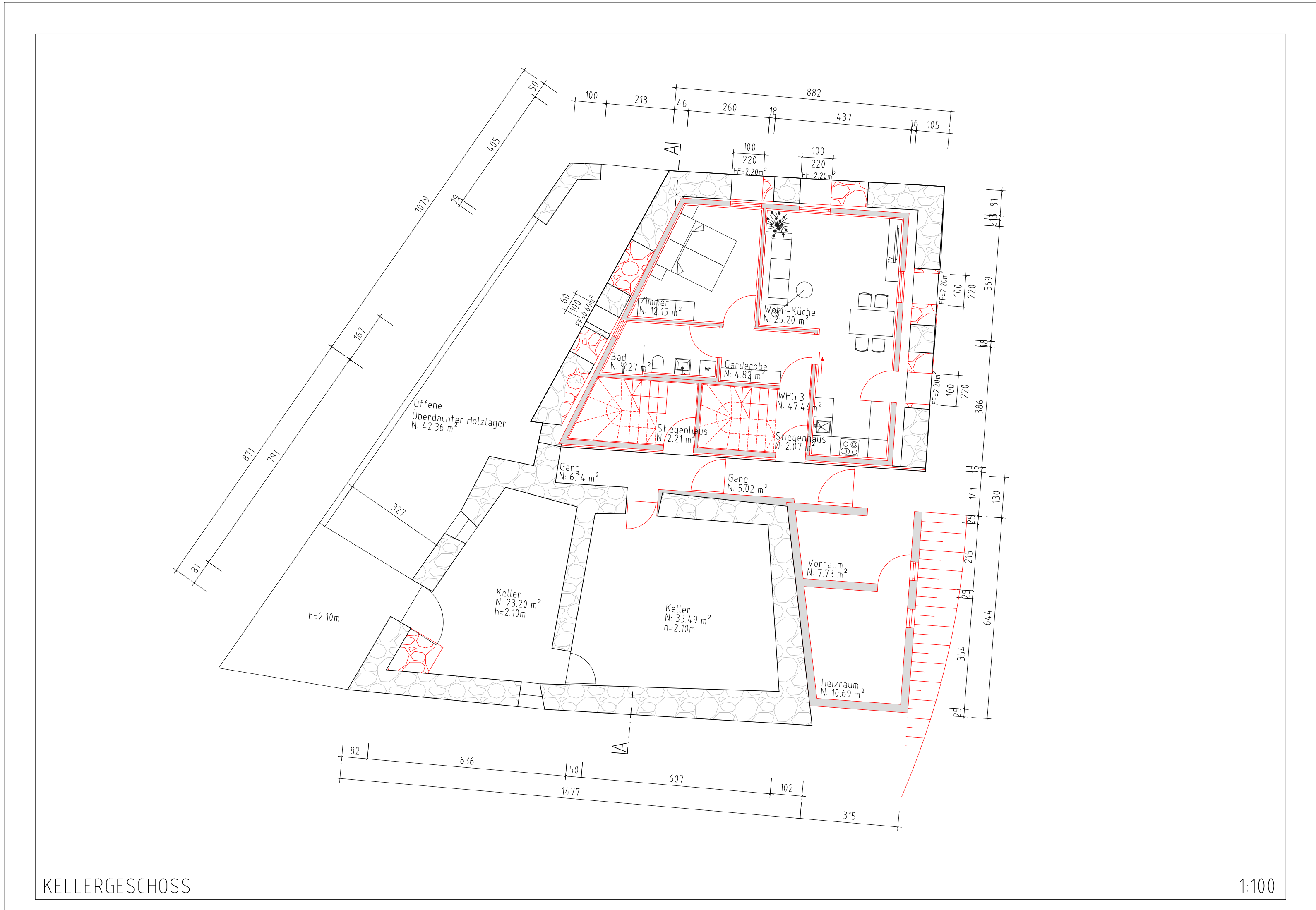
KELLERGESCHOSS
