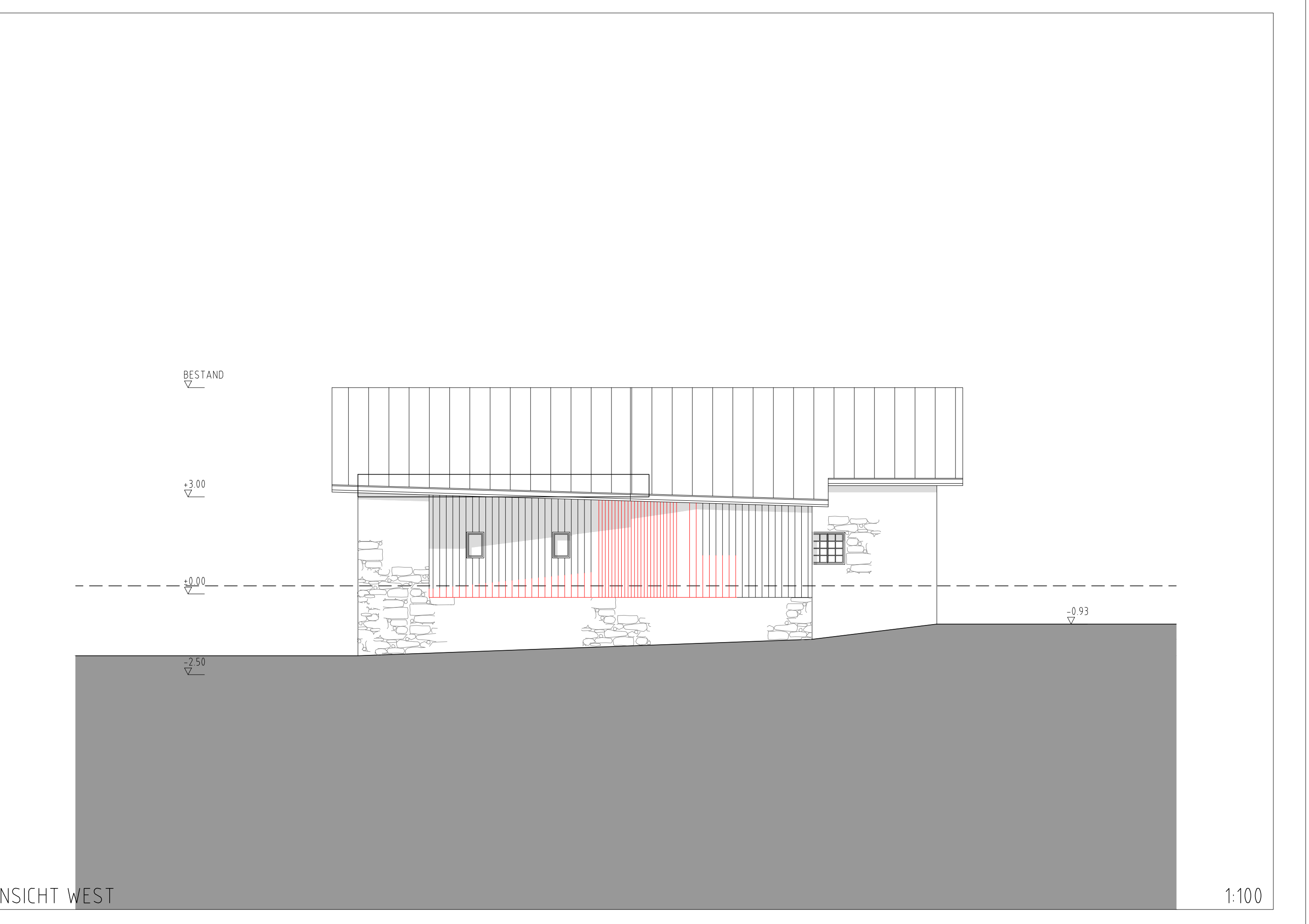
ANSICHT WEST
