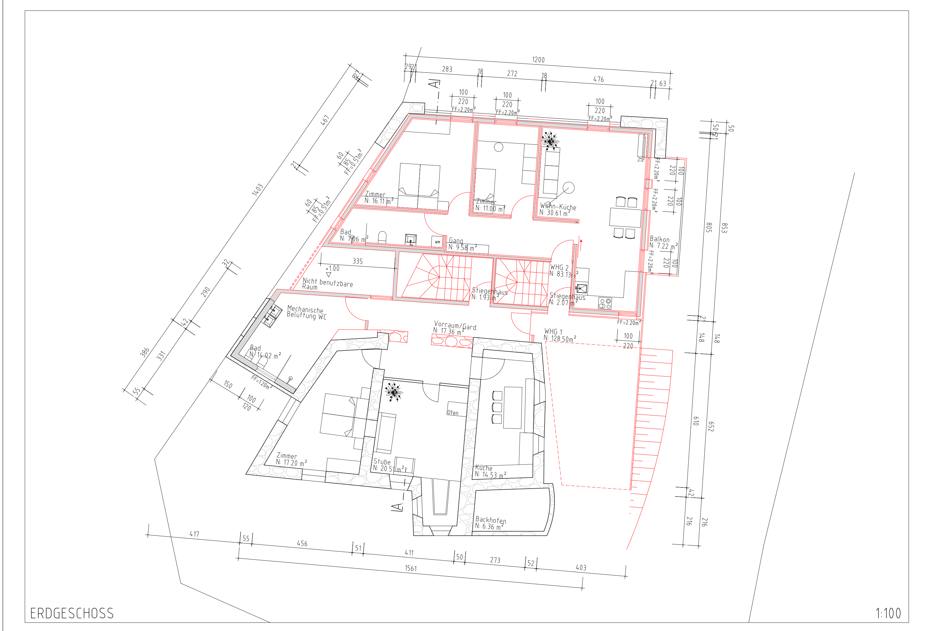
ERDGESCHOSS
