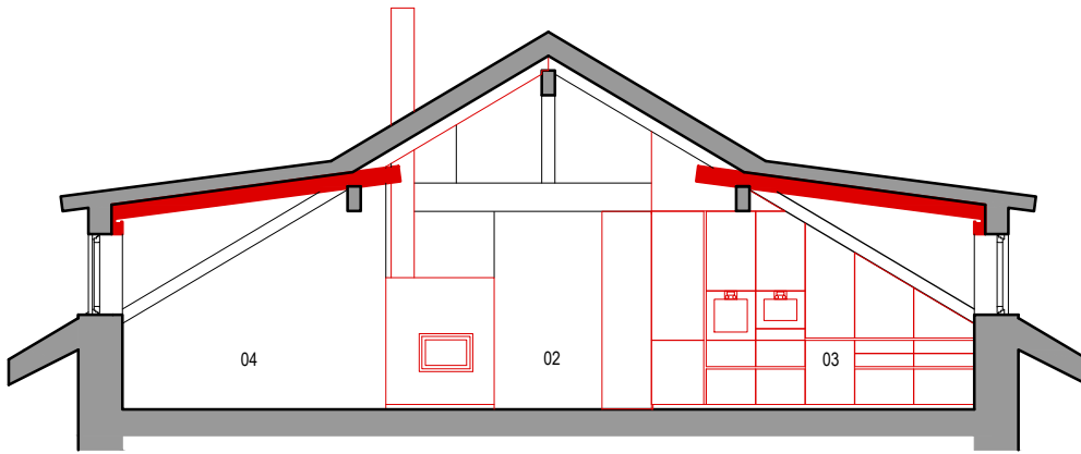
SCHNITT A-A_M.1:100
