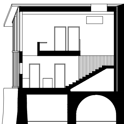
SCHNITT A-A
