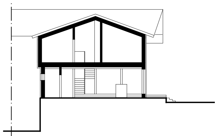
SCHNITT B-B
