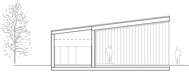
SCHNITT
