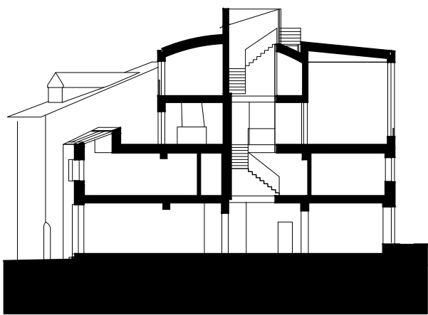
SCHNITT B-B / SEZIONE B-B
