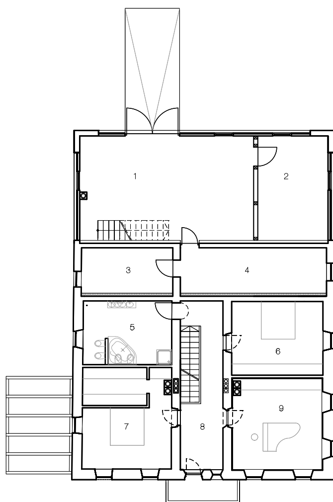
OBERGESCHOSS
