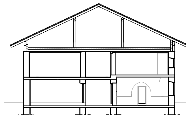
SCHNITT
