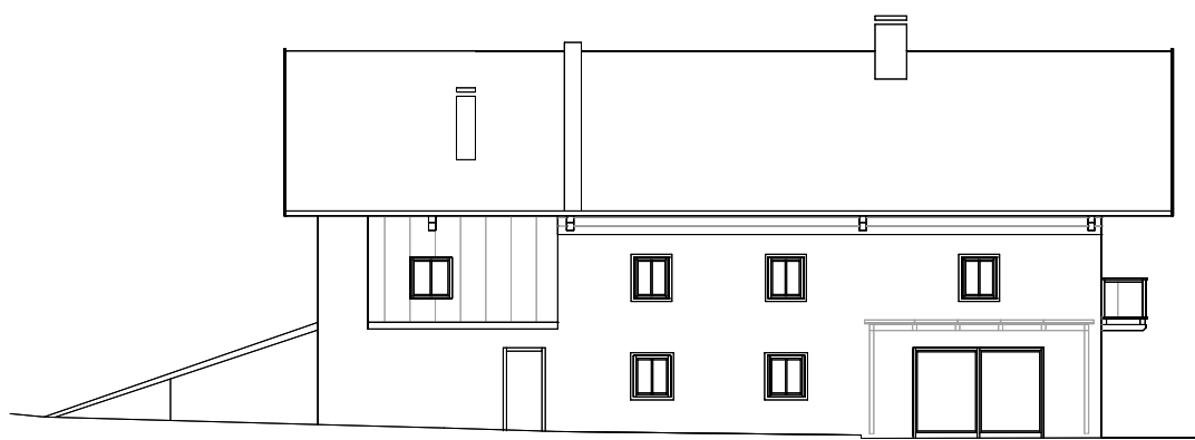
WESTANSICHT
