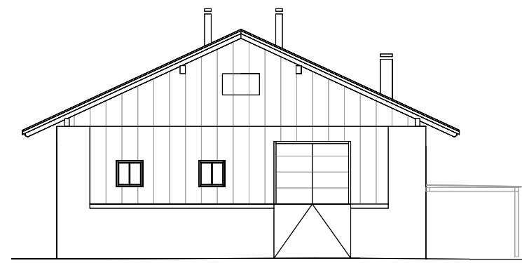
NORDANSICHT
