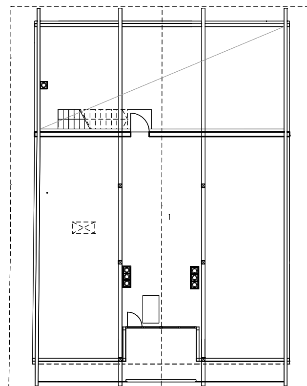
DACHGESCHOSS
